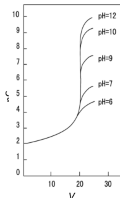
图 E5-2 不同 pH 下, 0.01000mol·L -1 EDTA 滴定 20.00mL 0.01000mol·L -1 Ca 2+ 的滴定曲线
