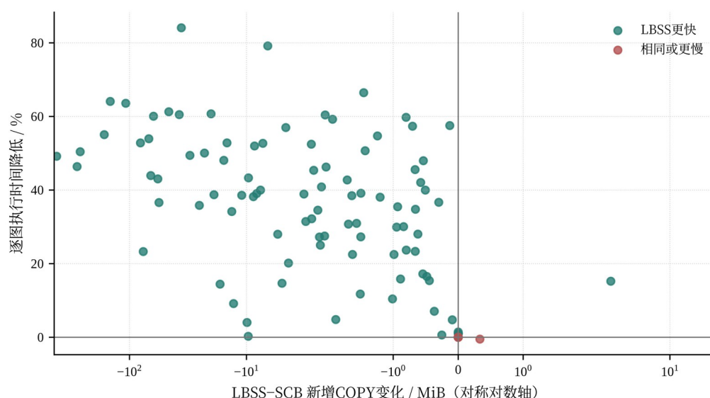
图 6-11 五核 B：执行时间与 COPY 的权衡
