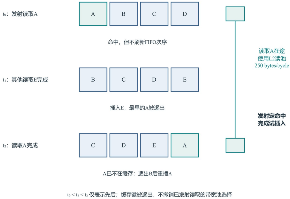
图 7-1 FIFO 状态快照与在途读取（示意图）
