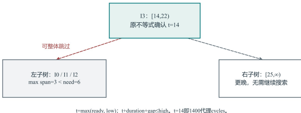
图 5-3 Treap 区间索引：相同插入规则，更少无效搜索（示意图）
