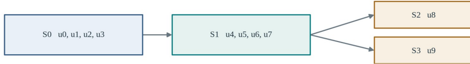
(c) 子图结果：带内按弱连通分量合并，不把整带强行并为一个Task
