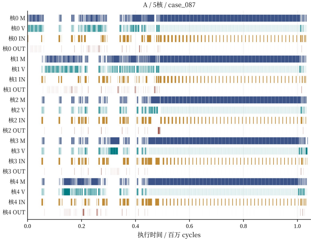
图 5-8 困难案例 case_087：五核执行时间线
