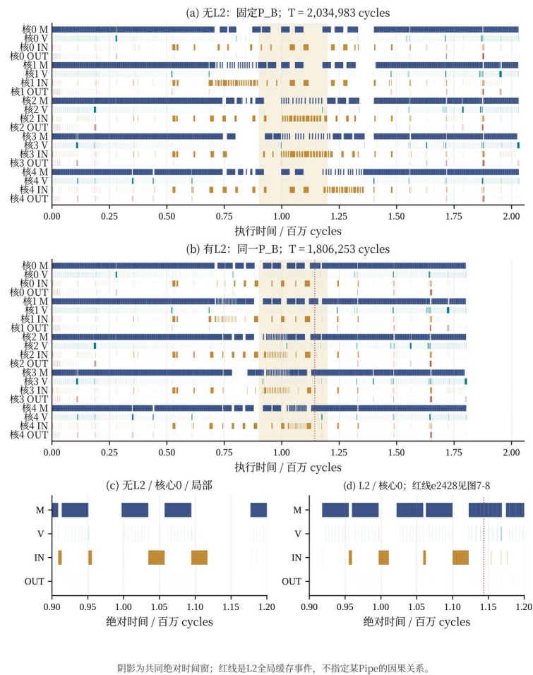
图 7-9 case_073: 同方案时间线与缓存事件定位
