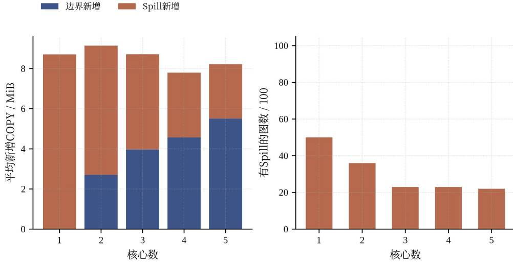
图 6-7 场景 B: 边界 COPY 与 Spill 分解
