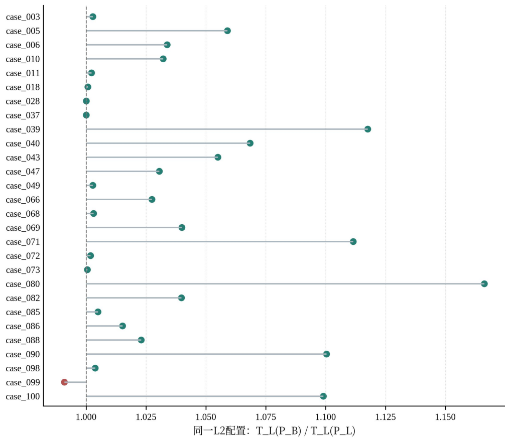
图 7-7 五核：不同最终方案的选择解效应
