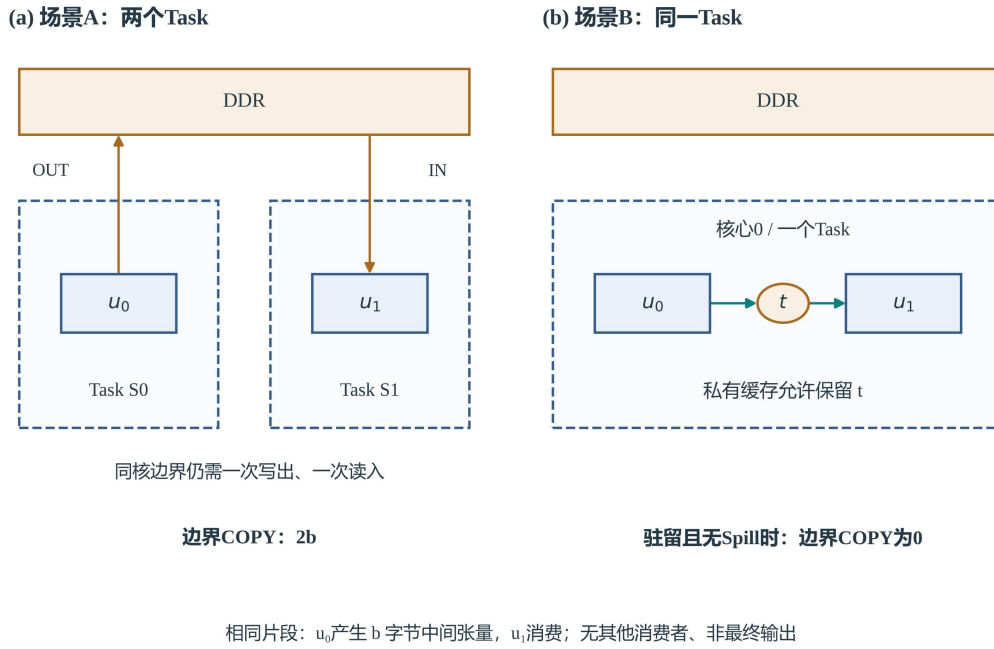
图 6-1 同一计算片段在场景 A 与场景 B 下的 Task 边界（示意图）
