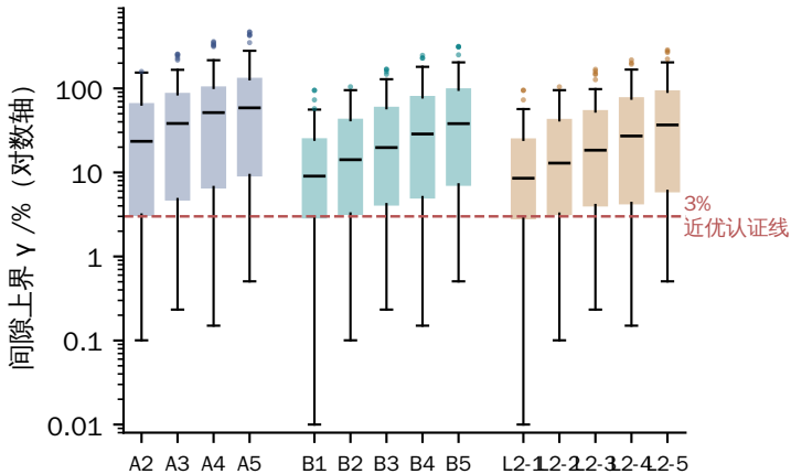
(a) 各场景、各核数的间隙上界分布
