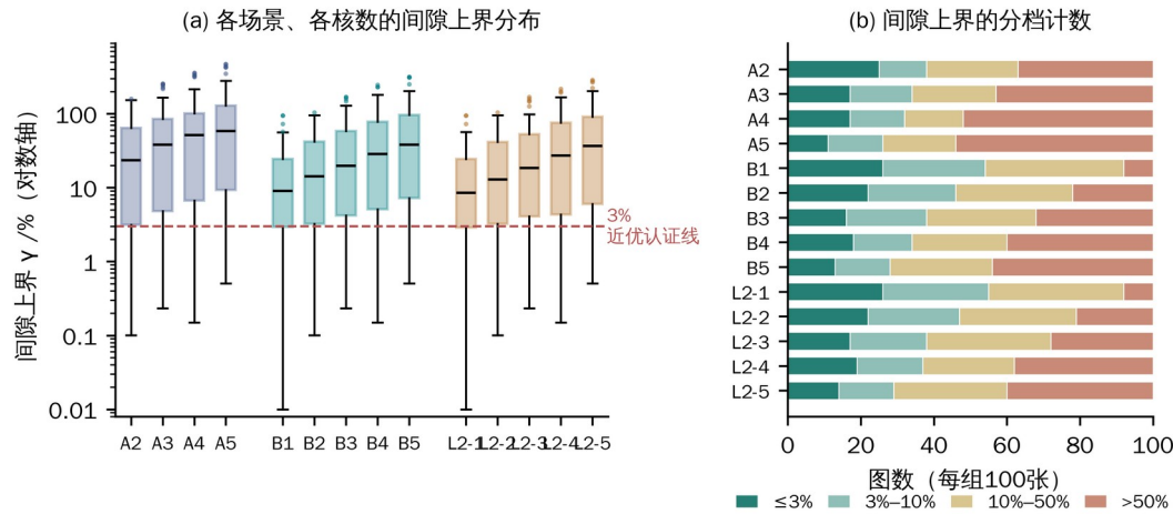
图 8-1 各场景、各核数的最优性间隙上界 \gamma 分布
