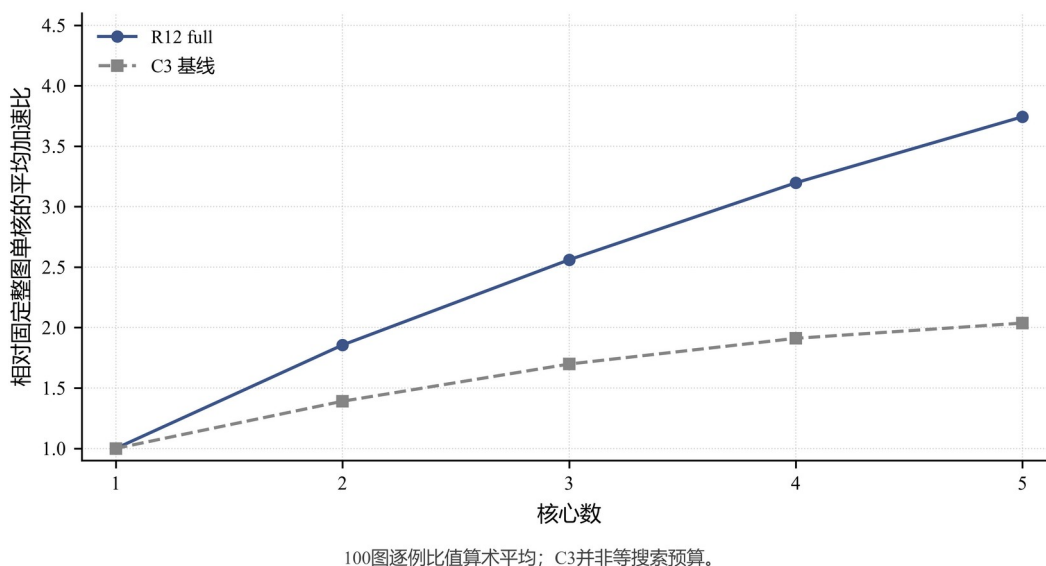
图 5-4 场景 A：核数扩展与参考性能
