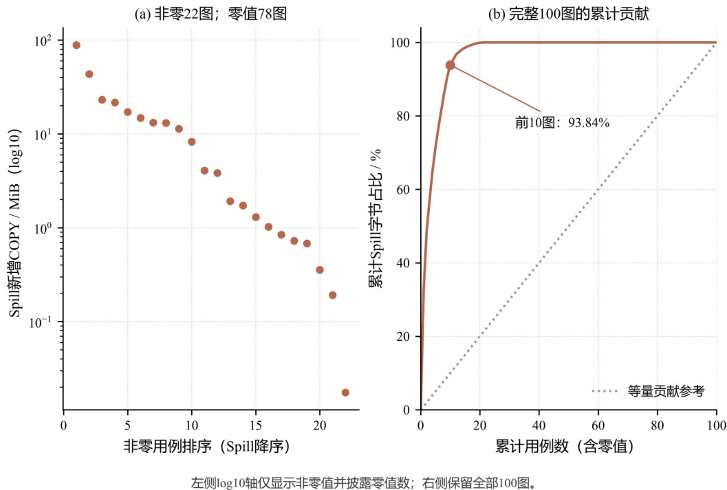
图 6-7 五核 B：非零 Spill 细节与全量集中度
