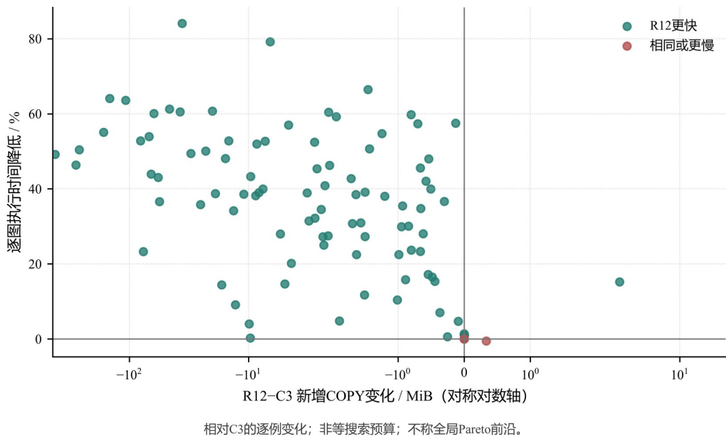
图 6-10 五核 B：执行时间与 COPY 的权衡
