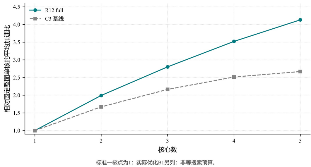
图 6-4 场景 B：核数扩展与参考性能
