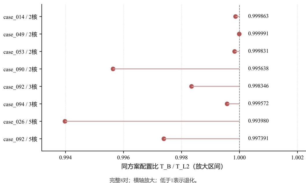
图 7-6 全部同方案 L2 退化记录
