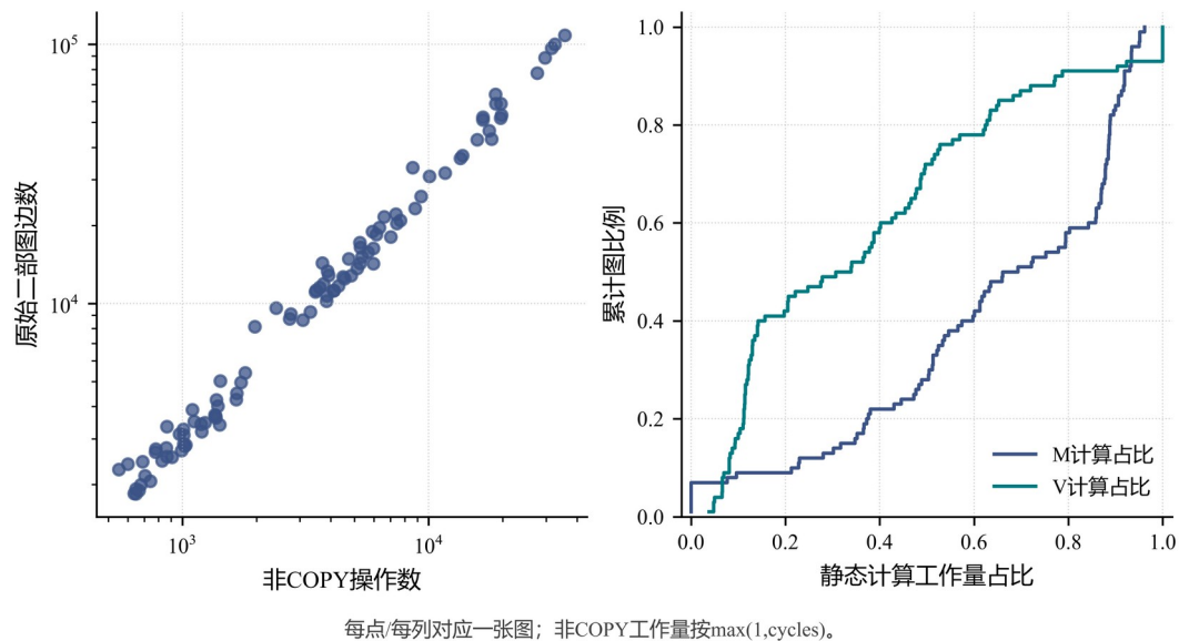
图 2-1 100 张计算图的规模与计算组成
