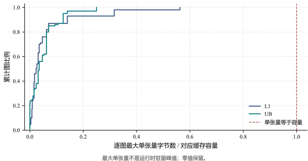
图 2-2 单张量大小与私有缓存容量
