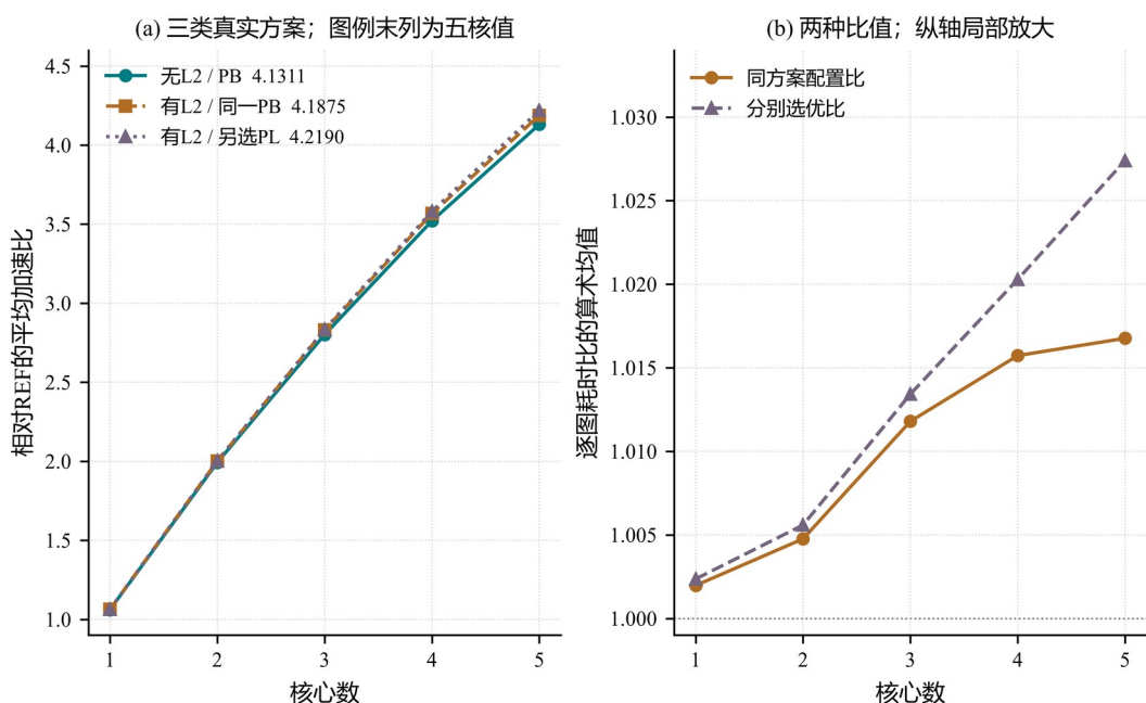
图 7-3 L2：三条方案曲线与两种配置比
