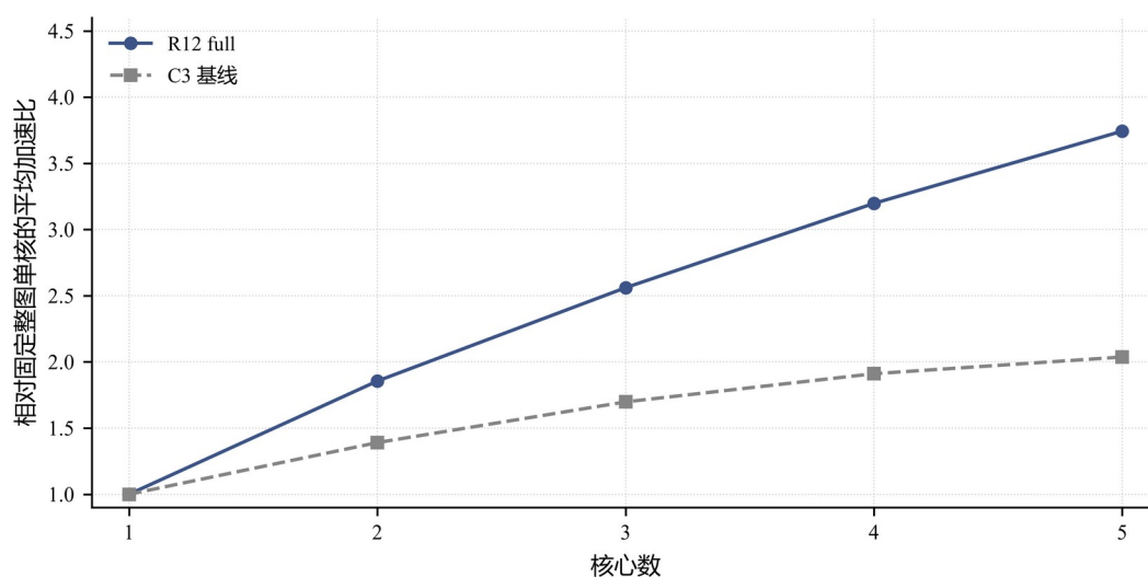
图 5-4 场景 A：核数扩展与参考性能
