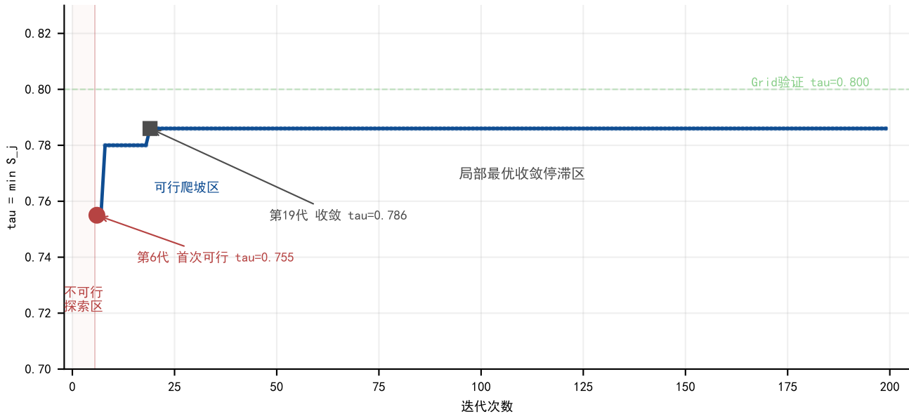
PSO收敛曲线 (Deb可行性规则, 100粒子, 200代)
