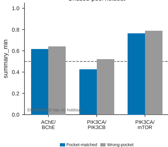
Unused-pool holdout
