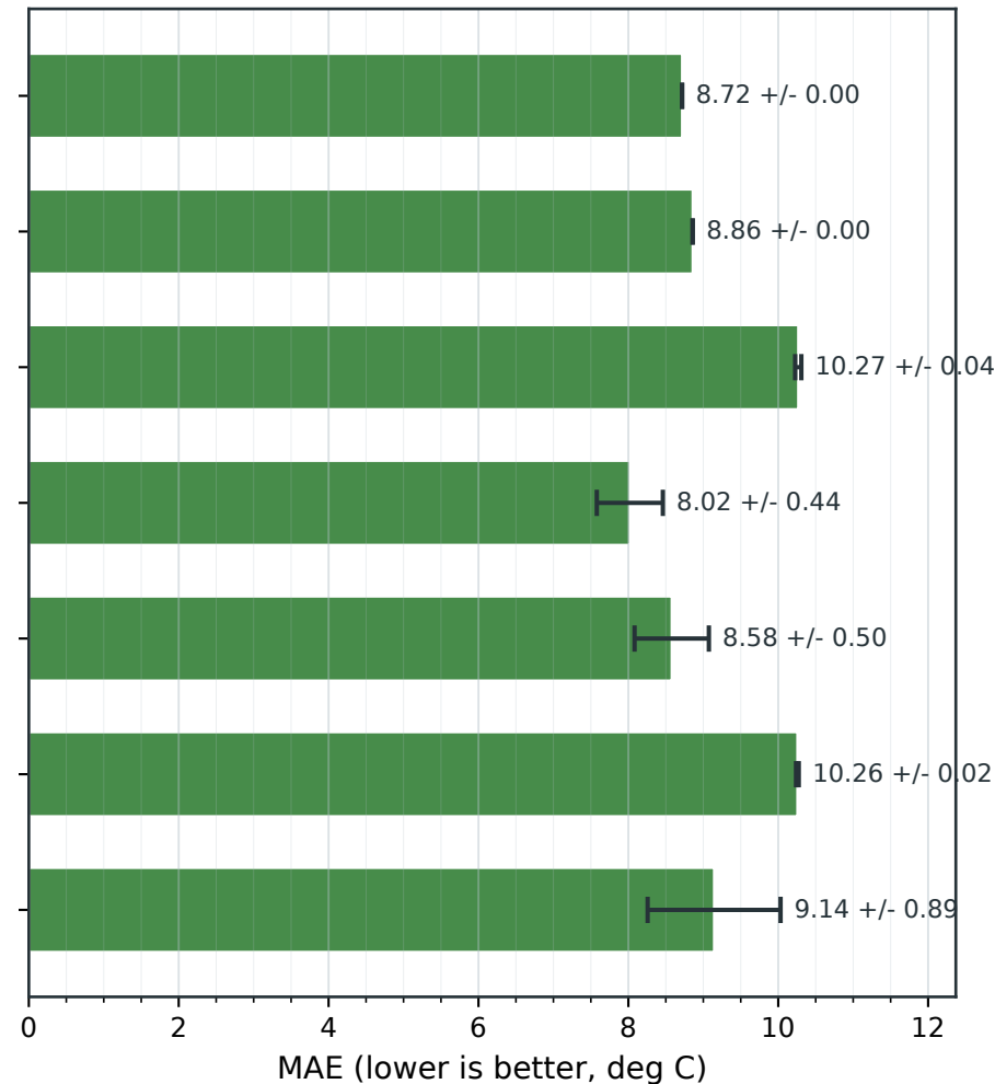
MAE
