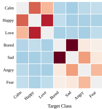
D2R
