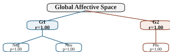
D2R: Vertical Hierarchy
