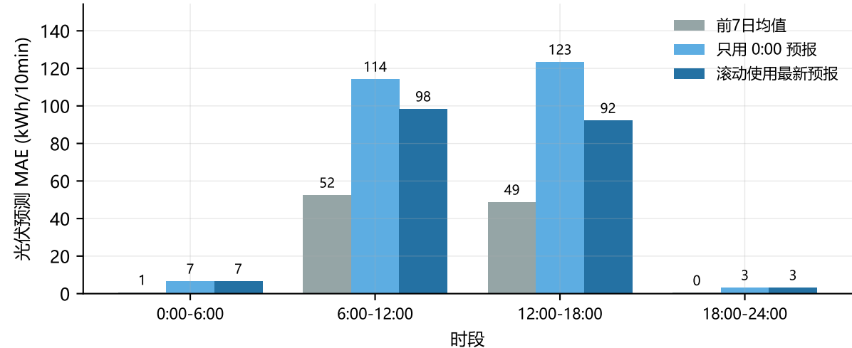
同一时段下三种光伏预测的误差对比
