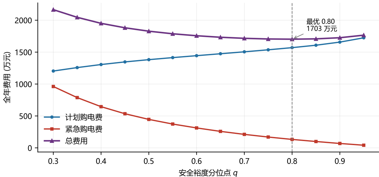
安全裕度取误差分布的 q 分位点时的问题2 全年费用
