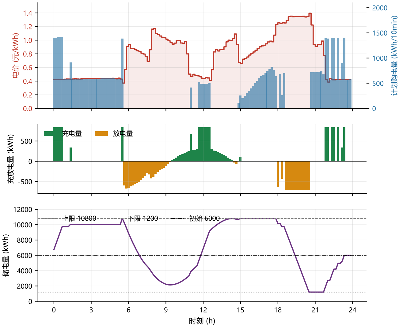
问题1 典型日：电价、购电量与储能调度
