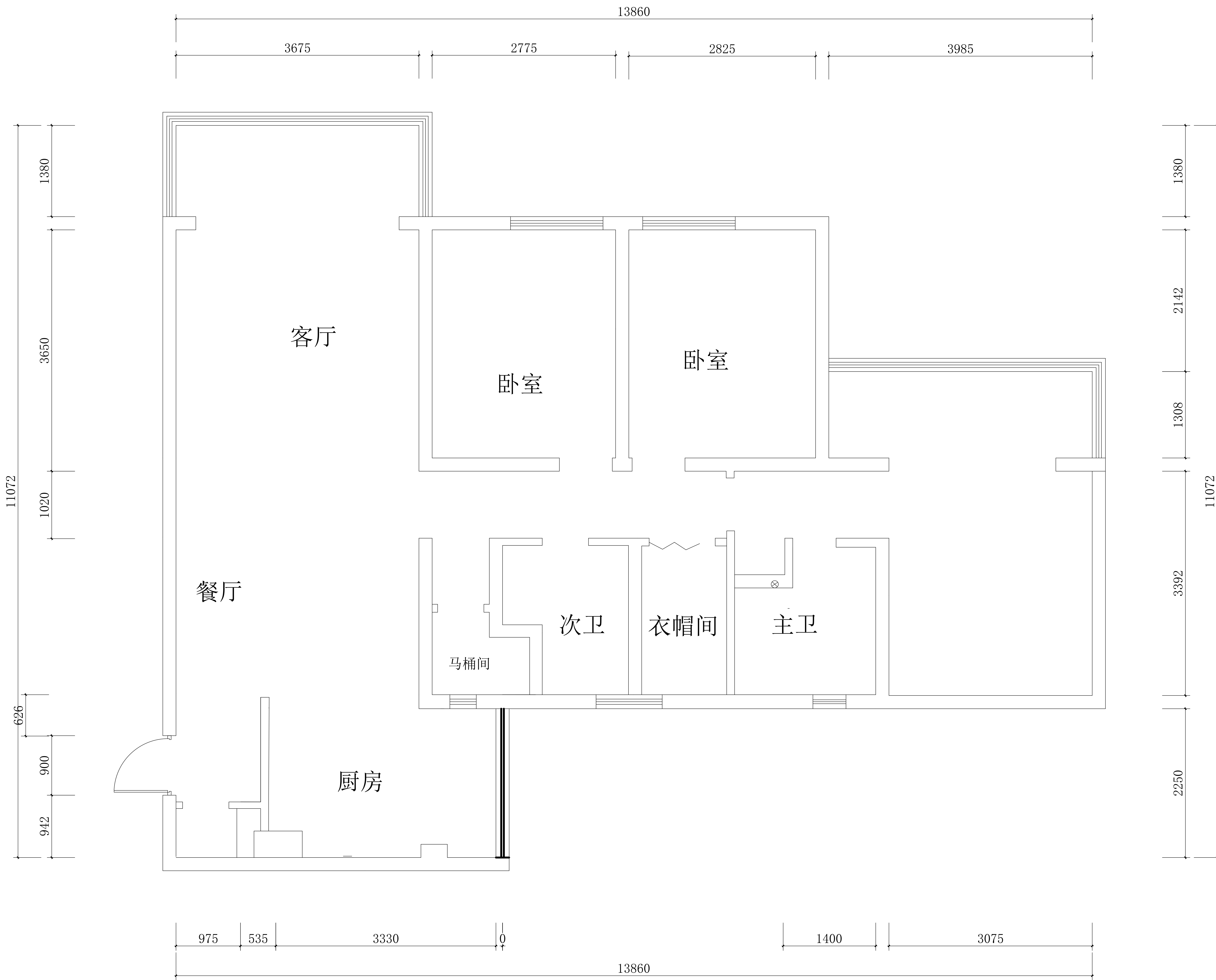
平面布置图
