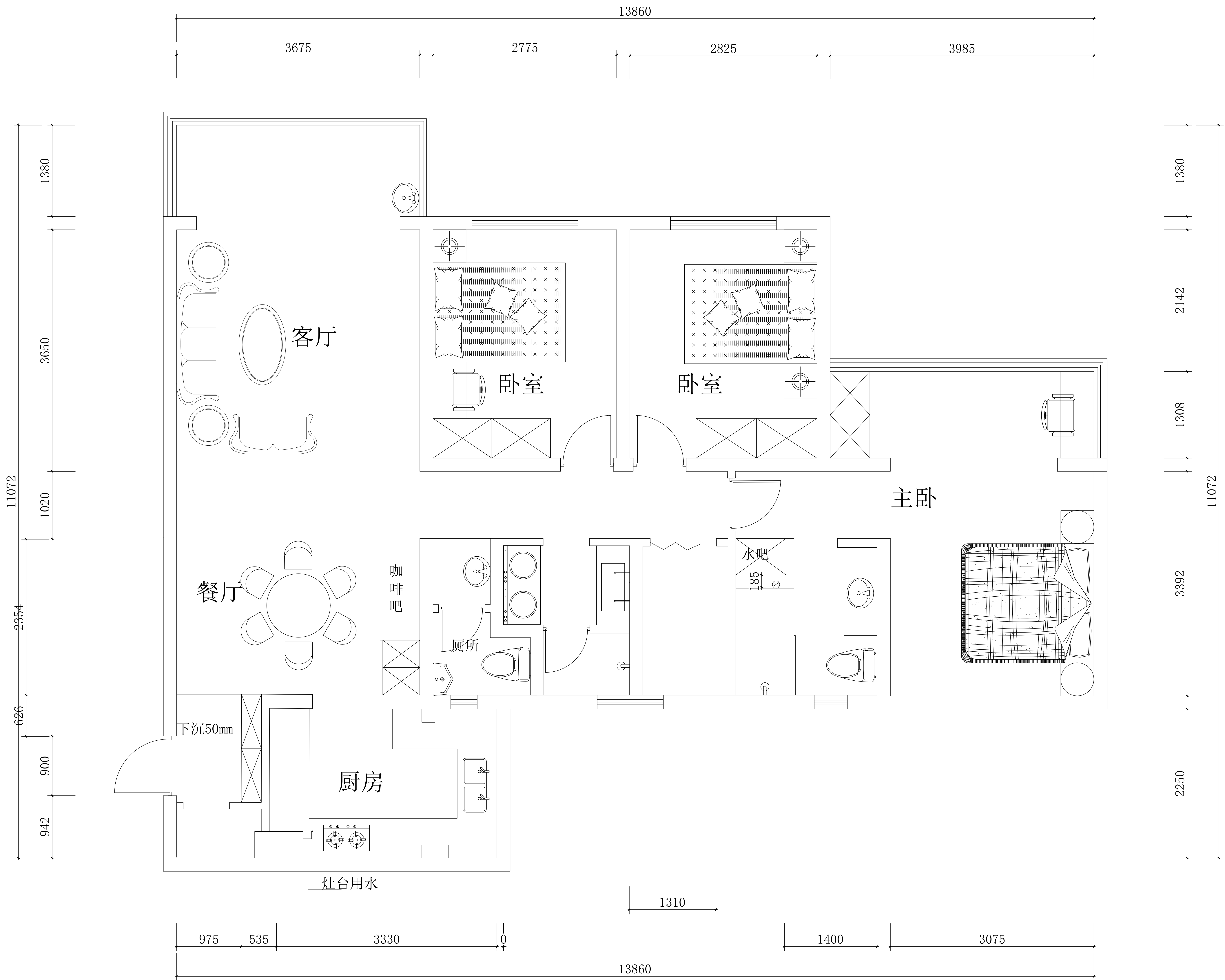
平面布置图
