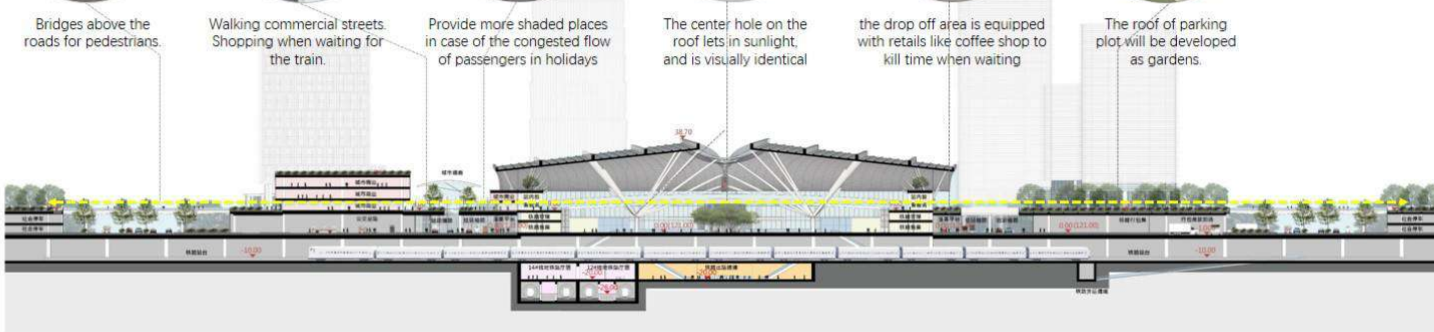
Section A-A'
