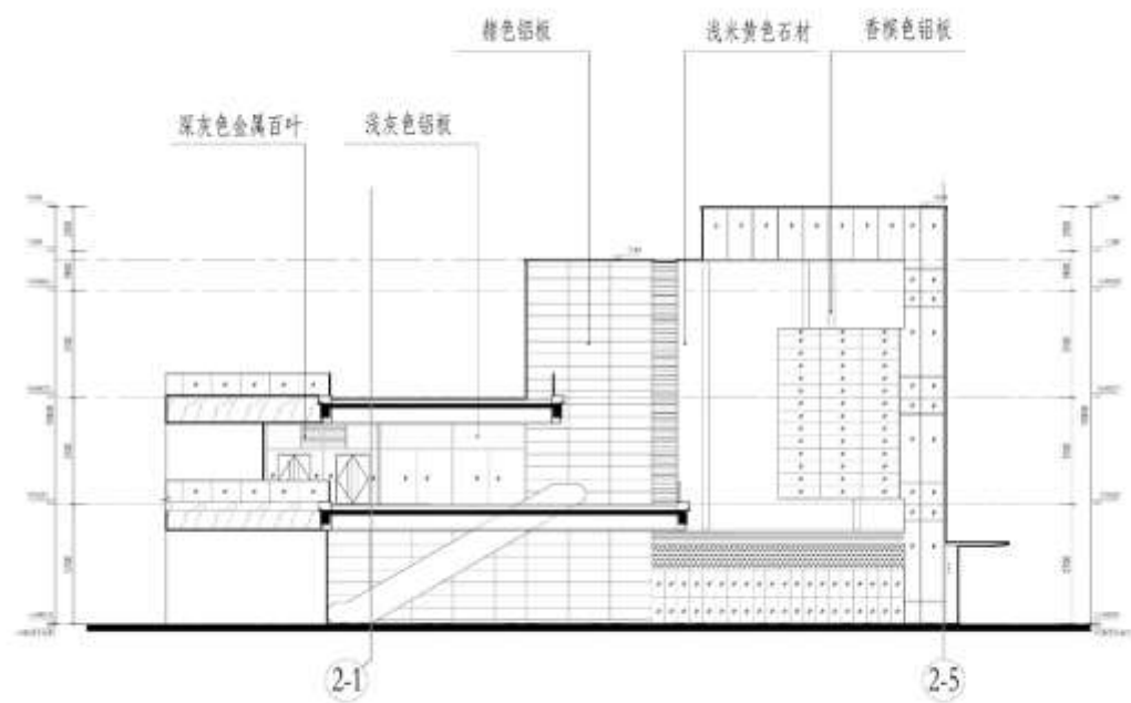
二号楼 01-05 轴(南)立面图 1: __
