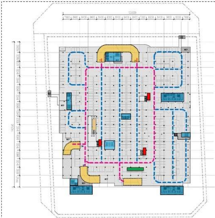
地下二层平面
