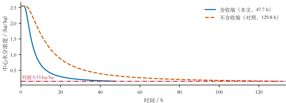
(b) 中心含水率：收缩把烘干时长压缩约 63%
