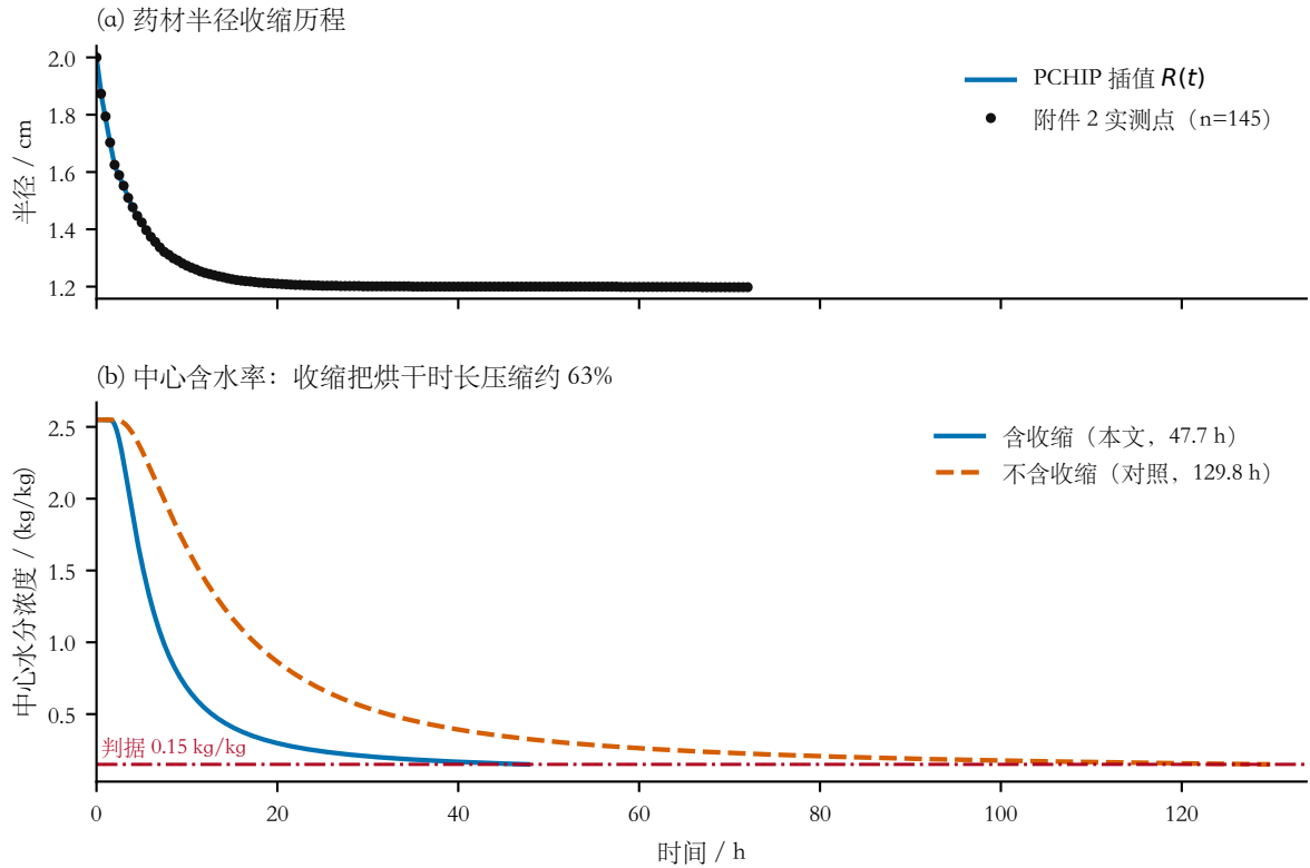
图 7 问题四：收缩历程与烘干时长的对照（附录 4 物性， N = 200 、 \Delta t = 5 s）。(a) 附件 2 的实测半径（ n = 145 ，间隔 1800 s，实测点以散点示出）与保单调三次 Hermite 插值曲线；插值后 \dot{R} \leq 0 恒成立、无过冲。(b) 中心水分浓度随时间的变化：含收缩时 47.73 h 达标，固定半径的对照工况需 129.79 h，收缩使烘干时长缩短约 63%。两图均为确定性数值结果，不含统计误差。
