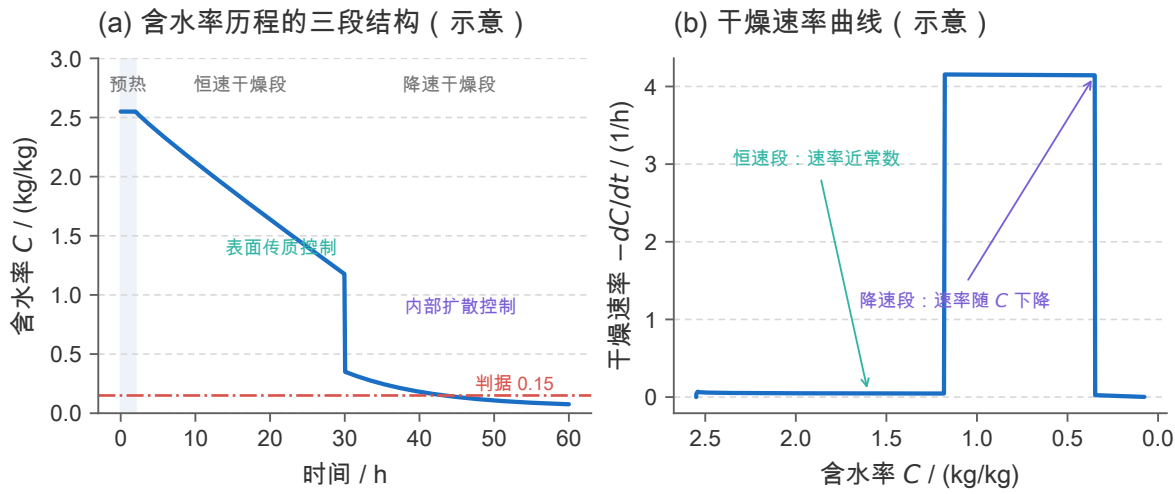
图 28 干燥三阶段的示意（用于说明概念，不是计算结果）。(a) 含水率历程按“预热平衡 → 恒速干燥 → 降速干燥”三段划分，红色点划线为 0.15 kg/kg 判据；(b) 对应的干燥速率曲线：恒速段的速率近似常数，降速段的速率随含水率单调下降。本文的实际结果（图 32）中看不到恒速段平台，原因是题给的 D = 2.4 \times 10^{-3} e^{-0.45/C} e^{-3850/T} 使扩散系数随含水率指数衰减，表面传质从未成为限制环节——这正是本题区别于经典恒速干燥的一个特点。
