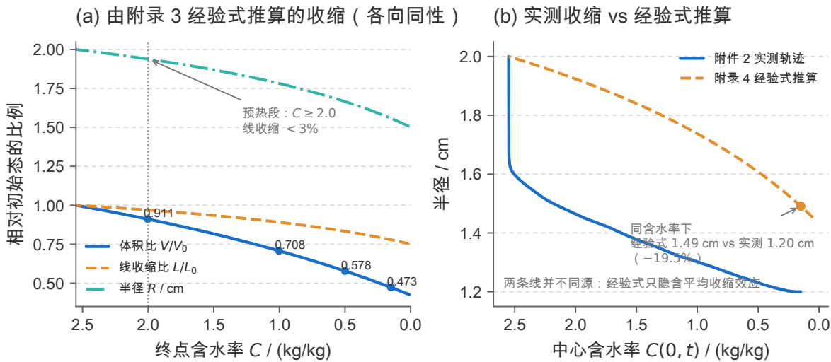
图 40 (a) 由附录 3 经验式推算的几何收缩: 体积比 V/V_0 、线收缩比 L/L_0 与对应半径随终点含水率的变化, 标注了正文四个报数点的数值; C \geq 2.0 时线收缩不足 3%。(b) 附录 4 经验式推算的 R(C) 与附件 2 实测 R-C 轨迹的对照, 两者在同一末态含水率下相差约 -19.5\% 。
