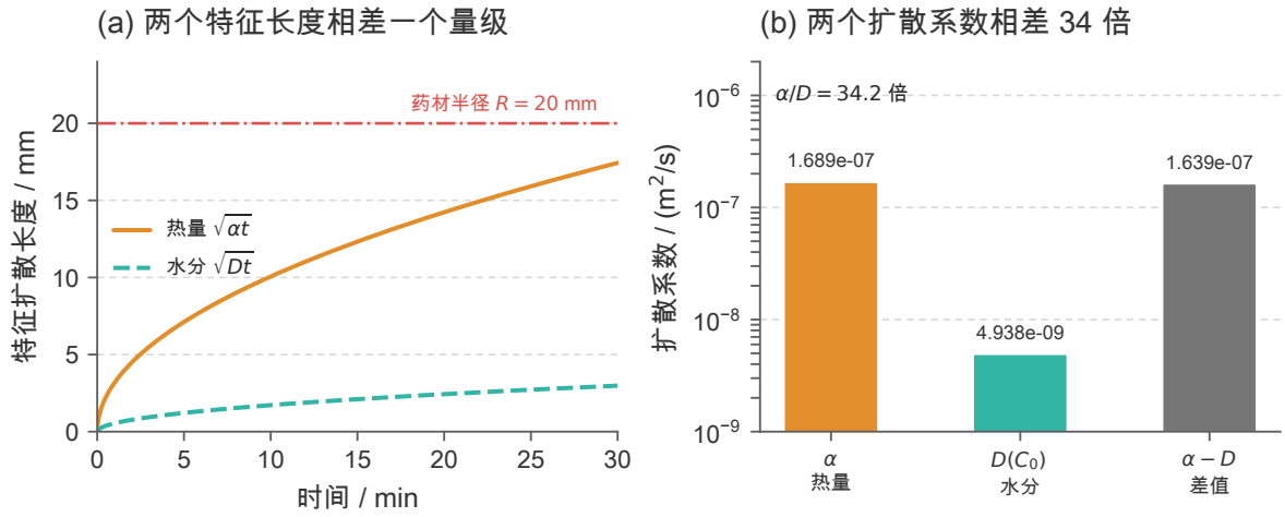
图 17 特征扩散长度与扩散系数的量级对比。(a) 热量的特征扩散长度 \sqrt{\alpha t} 与水分 \sqrt{D t} 随时间的变化：1800 s 时前者达 17.4 mm、已接近半径 R = 20 mm，后者仅 2.98 mm；(b) 两个扩散系数 \alpha = 1.689 \times 10^{-7} 与 D(C_0) = 4.938 \times 10^{-9} \text{ m}^2/\text{s} 相差 34.2 倍。两个数即可解释“温度全场重分布、水分只动最外 3 ~ 5 mm”，也说明表面传质阻力不是限制环节。
