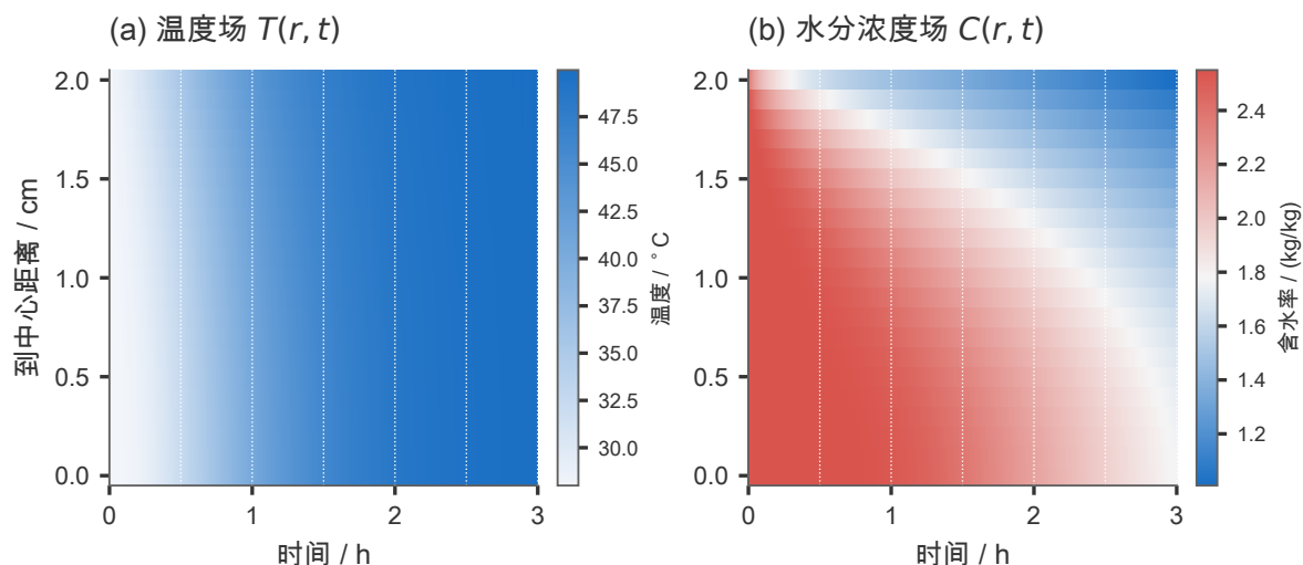
图 21 问题二 3 h 内两个场的时空演化。(a) 温度：等温线迅速变得近乎水平，说明温度场很快趋于准稳态；(b) 含水率：等值线是斜的，且干燥前沿随时间由表面向内部推进，全过程保持”外干内湿”的单调剖面。两图均为矩阵数据，采用感知均匀色图并附 colorbar，不构成”彩虹色图”式的误读。白色点线标出表 10、11 的报数时刻。
