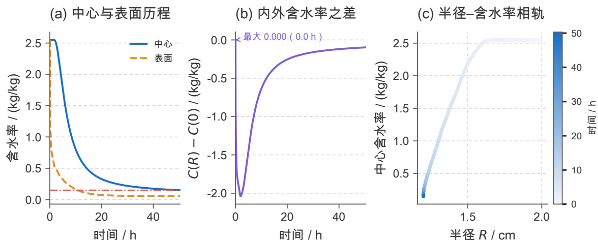
图 37 问题四的中心与表面历程。(a) 中心与表面含水率：两者始终相差一个可观量，且表面先达标；(b) 内外含水率之差 C(R) - C(0) （表面比中心干，故为负值）：其绝对值在 t \approx 2.0 h 达到最大 2.04 kg/kg，之后随整体趋于平衡而单调回落到约 0.10，说明干燥前沿在最剧烈收缩的阶段最深；(c) 半径-含水率相轨（颜色为时间），与图 5 同一含义，此处直接取自问题四的解，可看到半径在含水率还很高时就已经基本停止变化。
