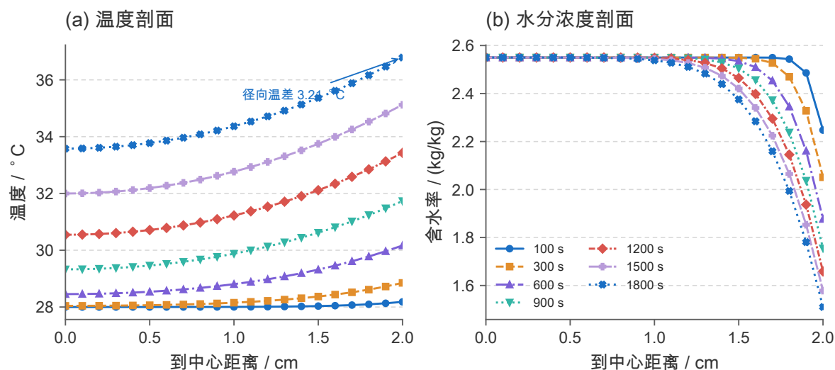
图 15 问题一各报数时刻的径向剖面（即表 7、8 的 100–1800 s 七行）。(a) 温度：整条剖面随时间整体抬升，且始终“外高内低”；(b) 水分浓度：0 ~ 1.0 cm 的曲线几乎完全重合，只有 1.5 cm 与 2.0 cm 处明显下降，直观印证“水分只动了最外侧 3 ~ 5 mm”。两图均采用线型 + 标记的双重编码，黑白打印时仍可分辨各时刻。
