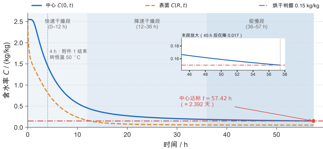
图 29 问题三干燥曲线：中心与表面水分浓度随时间的变化 ( N = 200 、 \Delta t = 5 s，判据为各点 C < 0.15 kg/kg)。红色点划线为烘干判据 0.15 kg/kg，阴影区依次为快速干燥段 (0-12 h)、降速干燥段 (12-36 h) 与极慢干燥段 (36-57.42 h)；后者耗时 21 h 却只换来 0.036 kg/kg 的下降。表面自 14.2 h 起即已达标 (占全程 23%)，全程由中心决定。竖向点线标出 4 h 处的阶段转换 (附件 1 结束、转入恒温 50^\circ\text{C} 工况)；右上角插图 of 45 h 之后的放大，把“最后 12 h 只降 0.017 ”这一反直觉结论直接呈现出来。
