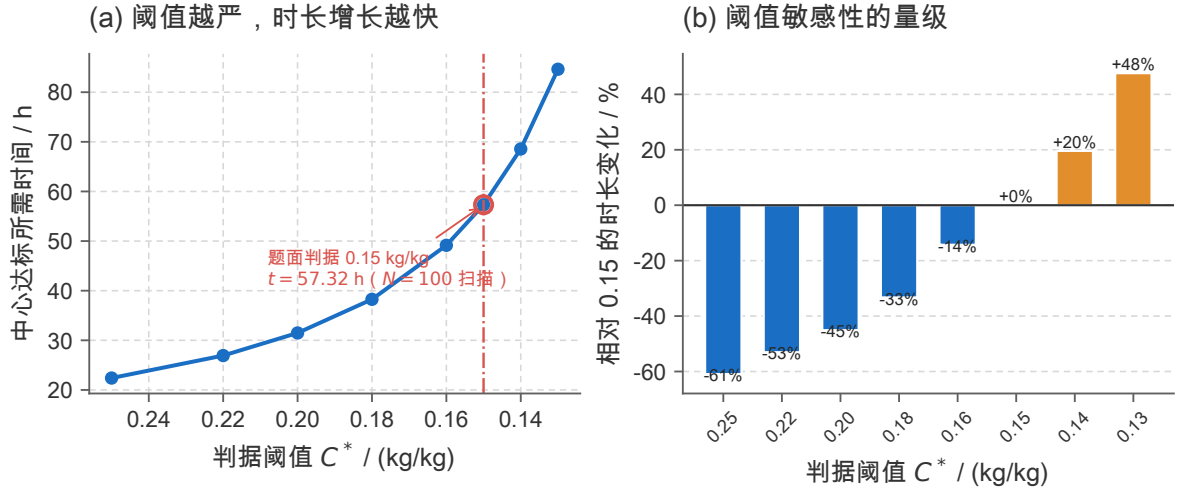
图 33 烘干判据阈值的敏感性 ( N = 100 、 \Delta t = 5 s 扫描)。(a) 中心达标所需时间随阈值的变化：阈值越严，所需时间增长越快，曲线在 C^* 低于 0.16 之后明显变陡；对应的烘干时长为 0.20 \rightarrow 31.5 h、0.18 \rightarrow 38.3 h、0.16 \rightarrow 49.2 h、0.15 \rightarrow 57.3 h、0.13 \rightarrow 84.6 h；(b) 相对题面判据 0.15 的时长变化率：把阈值放宽到 0.20 可省 45% 的时间，放宽到 0.25 可省 61%；而收紧到 0.13 则要多耗 48%。该图给出的是工艺建议的直接依据——在满足品质要求的前提下，判据每放宽 0.01 kg/kg 都能带来可观的时间与能耗收益，且这一结论比单点结果更能体现模型的稳健性。
