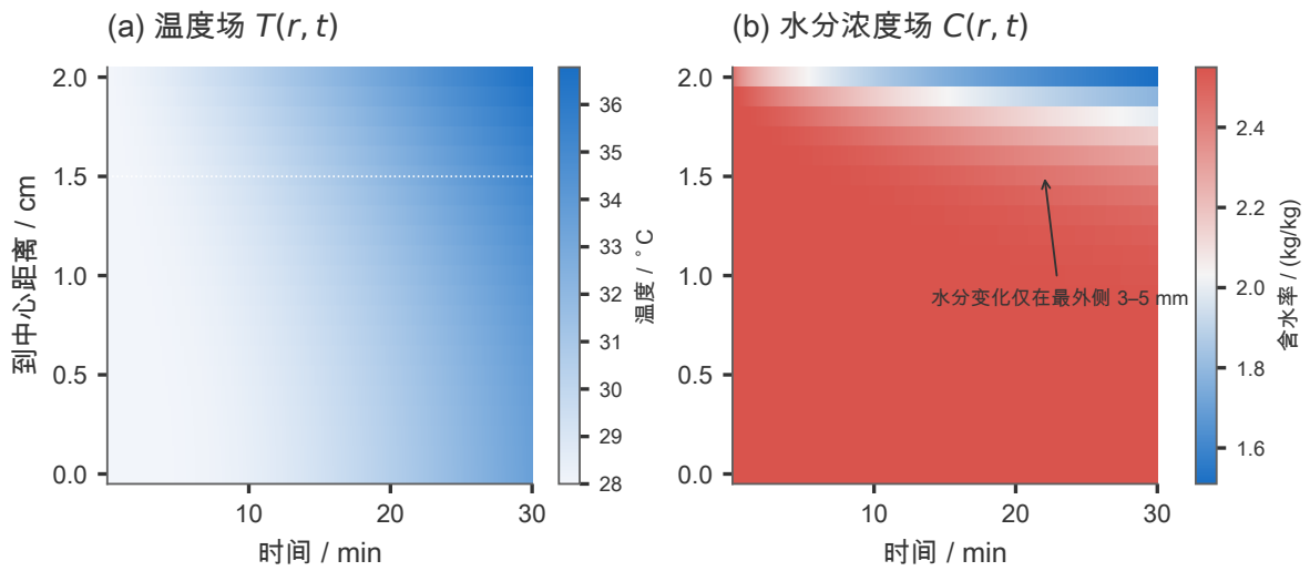
图 14 问题一温度场与水分浓度场的时空演化 (节点中心有限体积, N = 400 、 \Delta t = 1 \text{ s} , 图中纵轴为 21 个输出节点)。颜色即数值本身, 无色差含义。(a) 热量在 1800 s 内已传遍整个截面, t = 1800 \text{ s} 时中心 33.58^{\circ}\text{C} 、表面 36.79^{\circ}\text{C} ; (b) 水分变化被限制在最外侧约 3 ~ 5 mm 的薄层内, 中心含水率在四位小数内始终保持 2.5500 \text{kg/kg} 。
