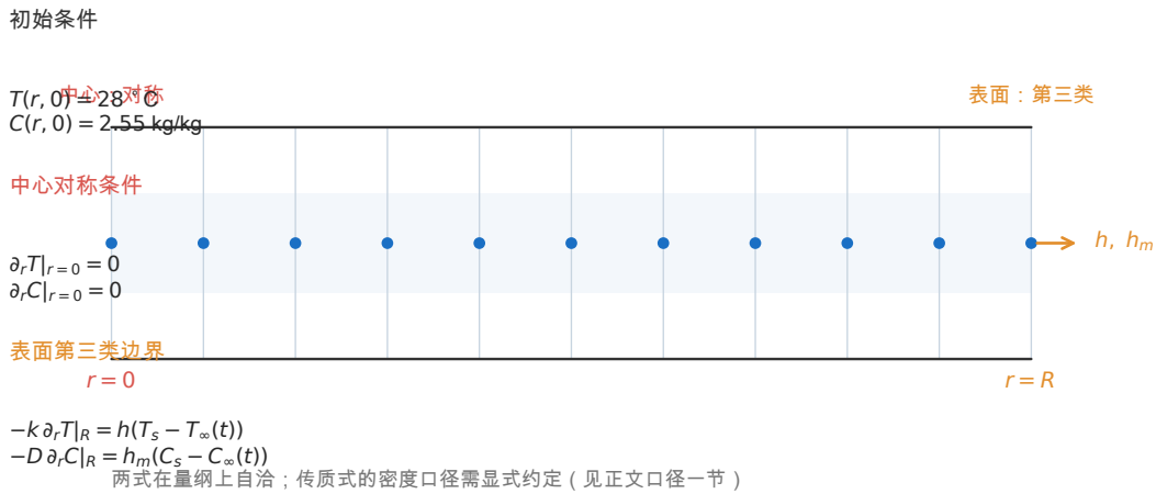
图 11 定解条件的构成（题面未给出，本文自建）。初始条件 T(r, 0) = 28^\circ \text{C} 、 C(r, 0) = 2.55 \text{ kg/kg} ；中心 r = 0 取轴对称条件 \partial_r T = \partial_r C = 0 ；表面 r = R 取第三类边界：换热由 h 驱动、传质由 h_m 驱动。两式在量纲上自治，但传质式的密度口径需要显式约定（见第 5.9 节）。
