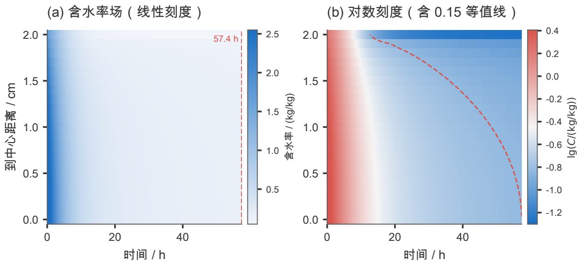
图 31 问题三全过程的含水率时空云图。(a) 线性色标：低含水率区间的层次被压得很扁；(b) 对数色标并叠加 C = 0.15 等值线（红虚线），可以清楚看到干燥前沿由表面向中心推进，等值线在 57.4h 才扫过中心轴。之所以并排给出两种色标，是因为判据附近的数值区间很窄，只有对数刻度才看得出层次；两图均附 colorbar 并标出单位。
