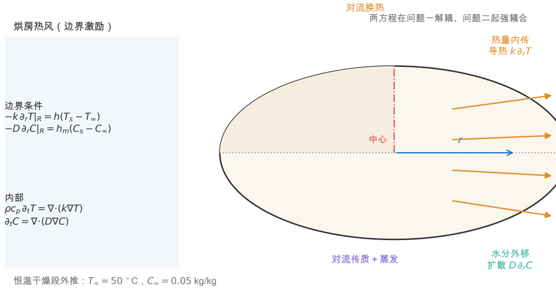
图 10 预热平衡阶段的物理图像与两条传输通道。烘房空气状态 T_\infty(t) 、 C_\infty(t) 是边界激励；药材内部温度由导热 k \partial_r T 向内传递，水分由扩散 D \partial_r C 向外迁移，两者在表面通过第三类边界与空气交换。左侧给出内部方程与表面边界条件，右上角点明本文的结构性结论：两个方程在问题一解耦、自问题二起强耦合。
