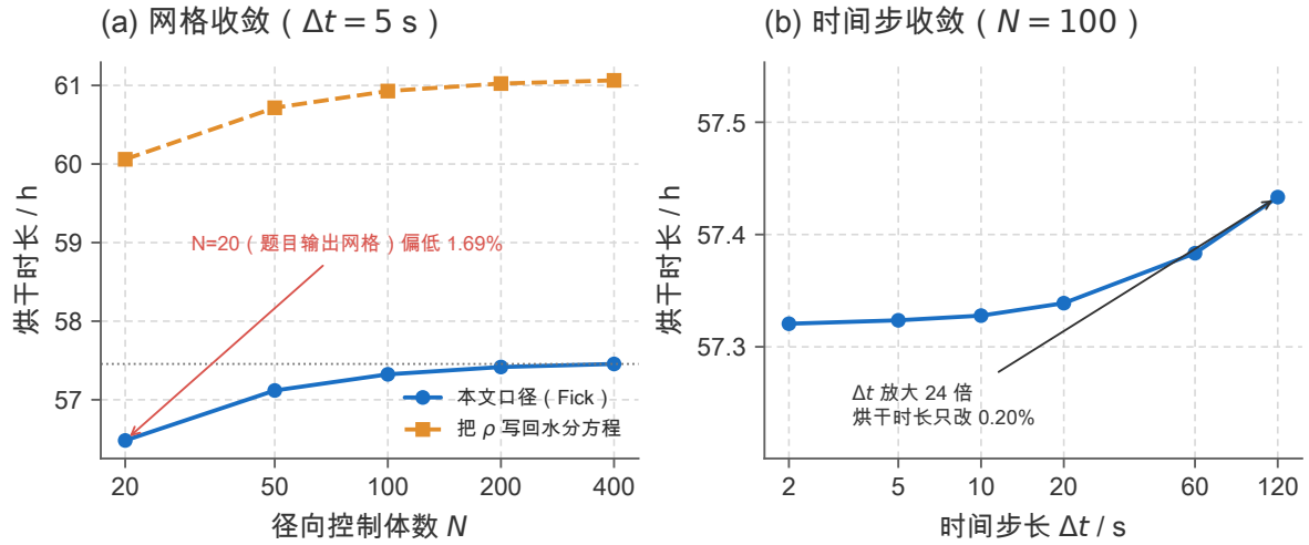
图 39 空间与时间离散的收敛性 (数据同表 17 与表 18)。(a) 固定 \Delta t = 5 \text{ s} , 改变径向控制体数 N : 本文口径与“把 \rho 写回水分方程”的变密度口径给出一对相互平行的收敛曲线, 说明口径差是模型层面的平移, 与网格无关; (b) 固定 N = 100 , 把时间步放大 24 倍, 烘干时长只改变 0.20%, 时间离散误差比空间离散小一个数量级。两图均为确定性计算, 不含统计误差。
