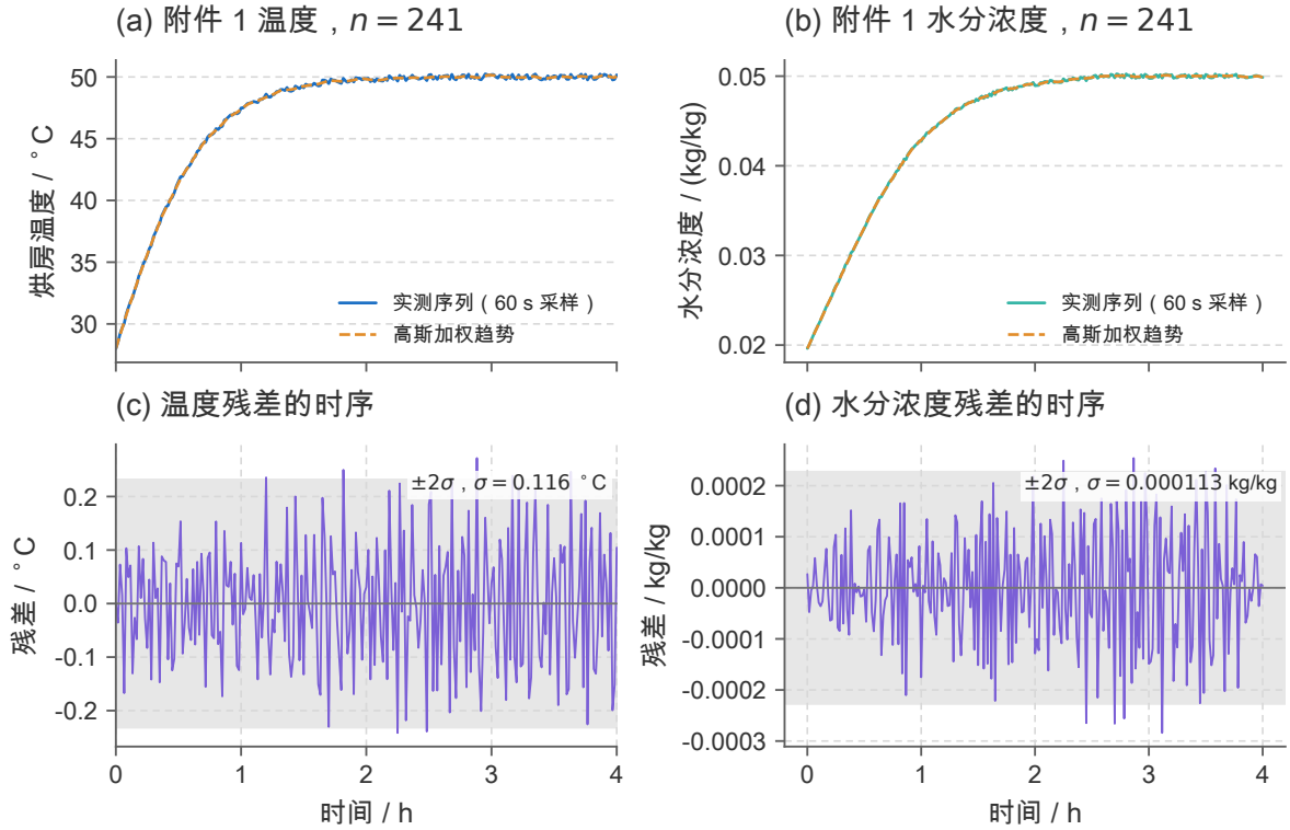
图 2 附件 1 实测序列与噪声诊断 ( n = 241 , 采样间隔 60\text{ s} )。 (a)(b) 烘房温度与水分浓度的实测序列 (实线) 与高斯加权局部二次趋势 (虚线, 窗口 15 点、无相位滞后); (c)(d) 两条序列相对各自趋势的残差, 灰色带为 \pm 2\sigma , 温度残差 \sigma = 0.116^{\circ}\text{C} 、水分浓度残差 \sigma = 1.1 \times 10^{-4} \text{ kg/kg} 。残差呈高频交替型 (滞后 1 自相关为负), 最大幅值仅约 2.3\sigma , 无异常点、无缺失。
