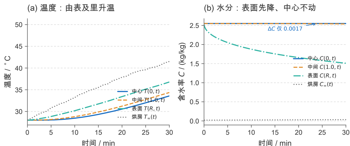
图 16 问题一中心 / 中间 / 表面与烘房状态的时间历程。(a) 温度：表面升温最快、中心最慢，30 min 内中心由 28.00 °C 升到 33.58 °C、表面升到 36.79 °C；(b) 水分浓度：表面由 2.5500 降到 1.5103，而中心在 30 min 内仅变化 0.0017。”温度全场重分布、水分只动表层”的对比是预热平衡阶段最本质的物理特征。
