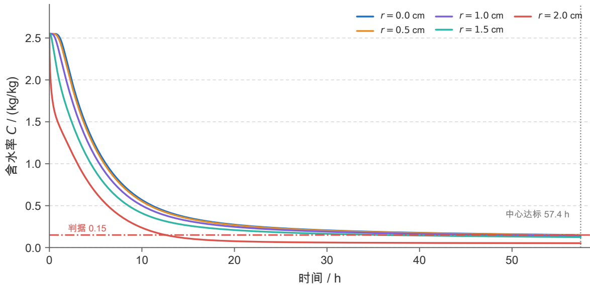
图 30 问题三各径向位置的含水率历程族 ( r = 0, 0.5, 1.0, 1.5, 2.0 cm)。五条曲线在 10 h 之前彼此分离，之后逐渐收拢并长期并行下降；最外层的 2.0 cm 曲线最早穿越判据 (约 14.2 h)，中心 0 cm 最晚 (57.42 h)。判据的控制点始终是中心，这正是把“各处达标”等价于 C(0, t) < 0.15 的图形依据。
