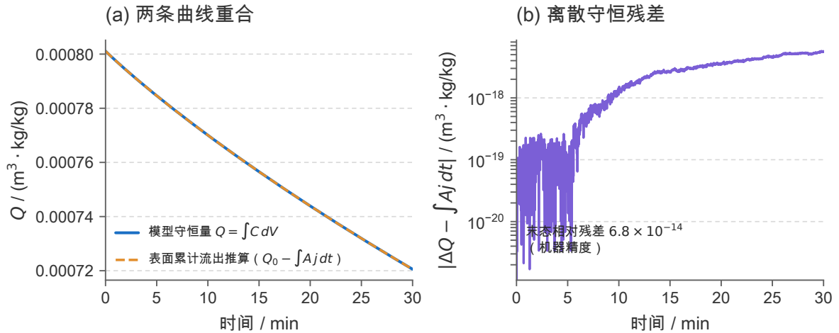
图 18 问题一的离散守恒性检验。(a) 模型守恒量 Q = \int C dV 的下降曲线与由表面累计通量 \int A_j dt 反推的曲线完全重合；(b) 两者之差（对数纵轴）始终处于机器精度量级，1800 s 末态的相对残差为 6.8 \times 10^{-14} 。需要强调守恒量应是 \int C dV 而不是 \int \rho_d C dV ——在本文采用的经典 Fick 口径下密度已被约去。
