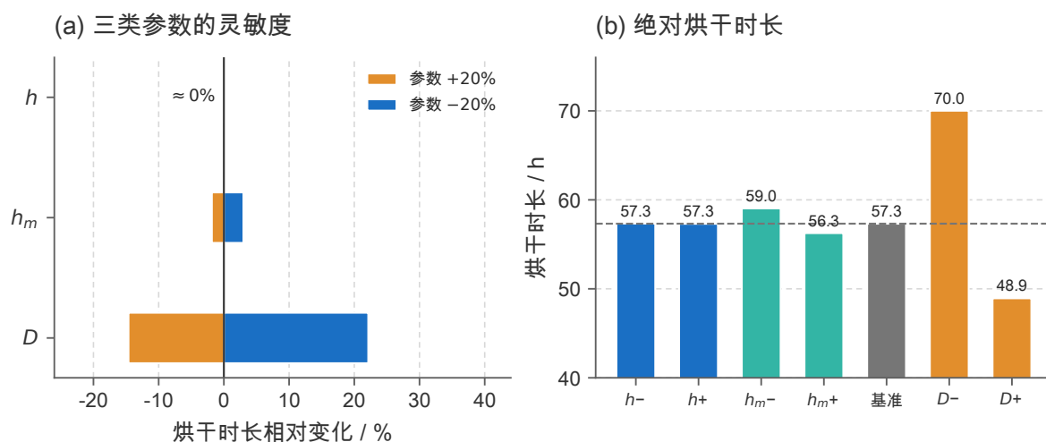
图 26 (a) 关键参数 \pm 20\% 扰动对问题三烘干时长的影响（基准 57.32 h， N = 100 、 \Delta t = 5 s，即表 17 与表 18 中的同一组设定）； h 的条形几乎为零宽，故直接标注 \approx 0\% 。(b) 各参数扰动工况的绝对烘干时长（灰色虚线为基准 57.32 h）： D 的扰动把时长拉到 48.9 ~ 70.0 h， h_m 只带来 56.3 ~ 59.0 h， h 几乎不动。该排序说明过程由内部水分扩散控制，表面换热阻力不是限制环节。两图均为确定性计算结果，不含统计误差，故不设误差棒。
