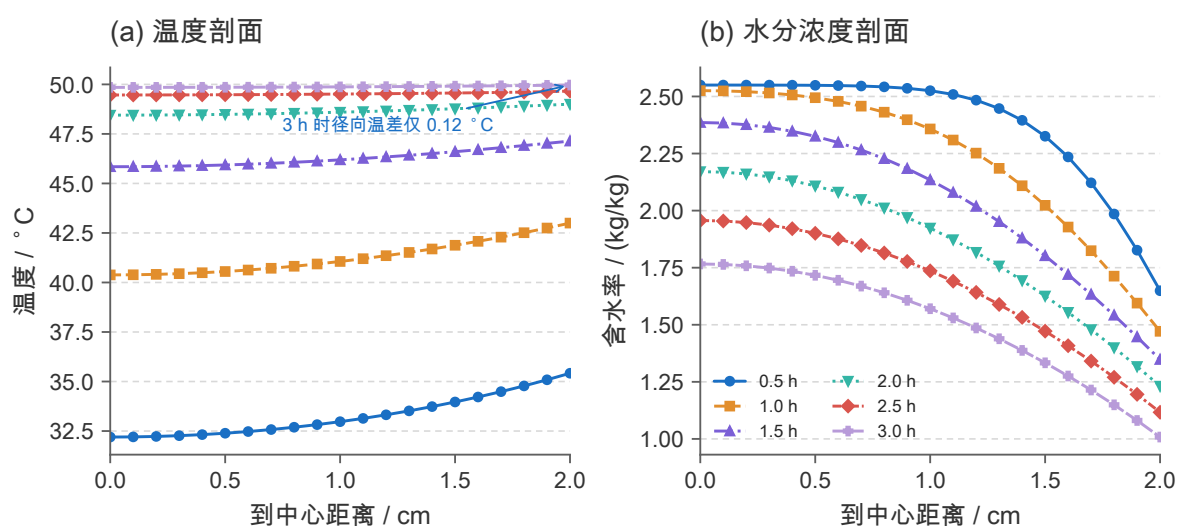
图 20 问题二 3 h 内温度与水分浓度的径向剖面（附录 3 变物性耦合模型， N = 200 、 \Delta t = 5 s，曲线取自 0 ~ 2.0 cm 等距 21 个输出节点）。6 条曲线分别对应 0.5、1.0、1.5、2.0、2.5、3.0 h，以线型与标记作冗余编码以适配色觉异常读者。(a) 2.5 h 后温度趋于均匀，3 h 时径向温差仅 0.12 °C；(b) 含水率始终保留由内向外的正梯度，说明过程由内部扩散控制。
