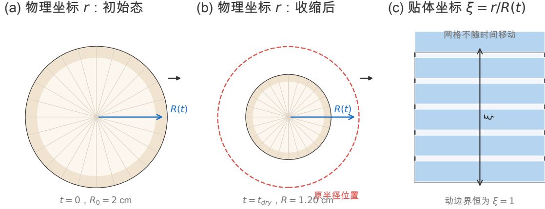
图 34 贴体坐标变换把动边界化为固定区域。(a) 物理坐标下 t = 0 的初始态，网格均匀铺在 r \in [0, R_0] 上；(b) 物理坐标下收缩后的状态，半径缩到 1.20 cm，若仍用固定物理网格，最外侧节点会落到药材之外；(c) 贴体坐标 \xi = r/R(t) 下动边界恒为 \xi = 1 ，网格不随时间移动，代价是方程中多出一个 \xi \dot{R} \partial C / \partial \xi 的对流项。这正是问题四与前三问在数值上的唯一结构性差别。
