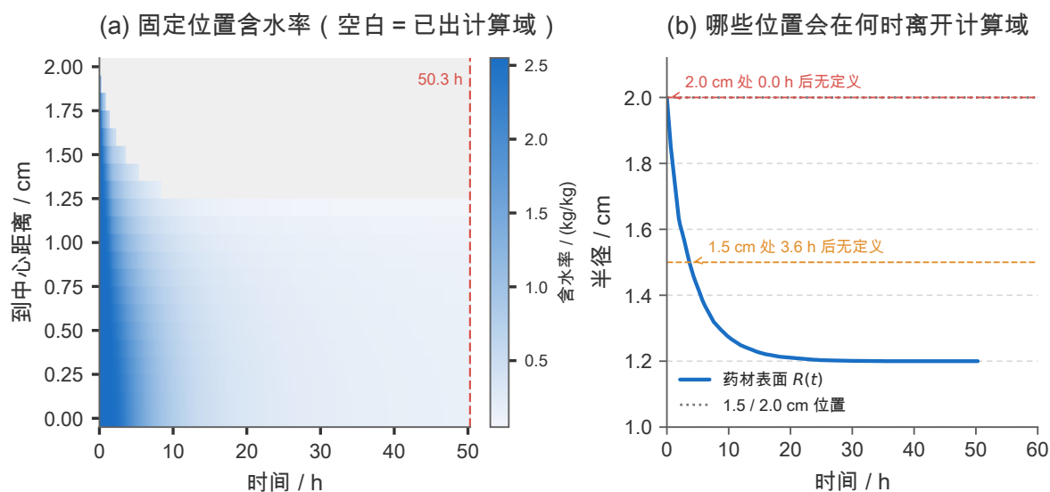
图 36 问题四的含水率时空场与计算域变化。(a) 在固定物理位置上给出的含水率云图：随着半径收缩，1.5 cm 与 2.0 cm 两列先后失去定义（图中灰色区域），这正是表 16 中以“——”表示的原因，也是题面模板允许留空的依据；(b) 药材表面 R(t) 与两条水平参考线的交点标出了“哪些位置会在何时离开计算域”：2.0 cm 处除初始时刻外均已越界，1.5 cm 处自 3.6 h 起无定义（1.0 cm 处始终在药材内部）。
