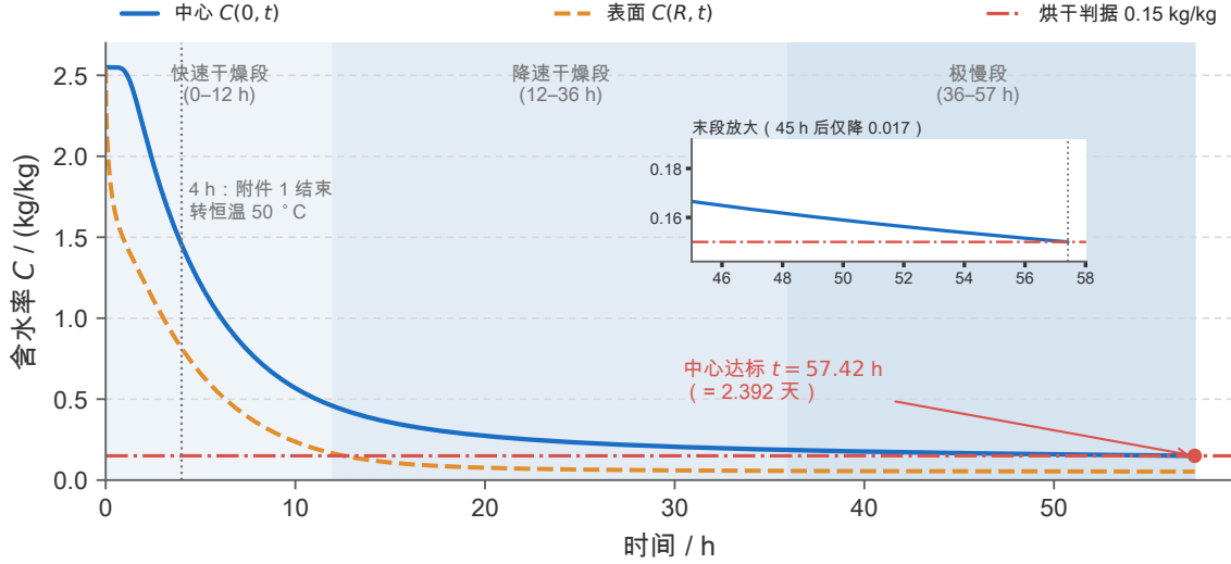
图 10 问题三干燥曲线：中心与表面水分浓度随时间的变化（ N = 200 、 \Delta t = 5 s，判据为各点 C < 0.15 kg/kg）。红色点划线为烘干判据 0.15 kg/kg，阴影区依次为快速干燥段（0–12 h）、降速干燥段（12–36 h）与极慢干燥段（36–57.42 h）；后者耗时 21 h 却只换来 0.036 kg/kg 的下降。表面自 12.6 h 起即已达标（占全程 22%），全程由中心决定。竖向点线标出 4 h 处的阶段转换（附件 1 结束、转入恒温 50 °C 工况）；右上角插图 of 45 h 之后的放大，把“最后 12 h 只降 0.017”这一反直觉结论直接呈现出来。
