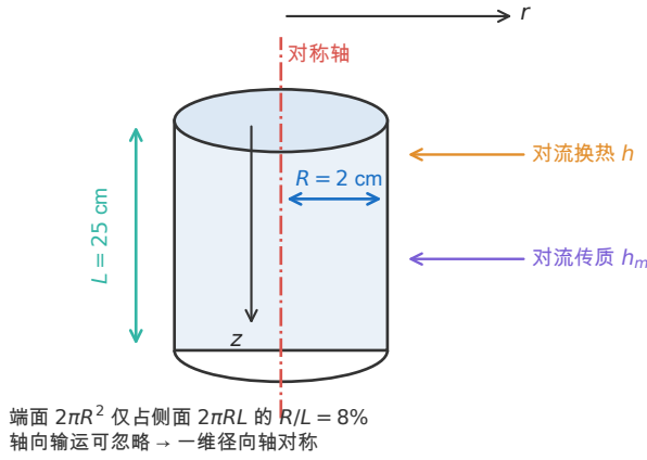
图5 圆柱形药材的几何、柱坐标与一维径向简化。(a) 几何与坐标架：药材长 L = 25\text{ cm} 、半径 R = 2\text{ cm} ，取柱坐标 (r, z) ， r 为到中心轴的距离、 z 为轴向；侧面同时发生对流换热 ( h ) 与对流传质 ( h_m )，端面面积 2\pi R^2 仅占侧面积 2\pi RL 的 R/L = 8\% ，故轴向输运可忽略。(b) 横截面上的简化：由轴对称性，场量与周向角无关，问题退化为一维径向问题 T(r, t) 、 C(r, t) ；中心 r = 0 为对称边界 ( \partial_r T = \partial_r C = 0 )，表面 r = R 为第三类边界；蓝色环状区域即后文有限体积离散所用的控制体 2\pi r dr dz 。
