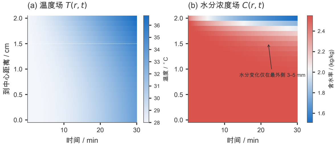
图 6 问题一温度场与水分浓度场的时空演化（节点中心有限体积， N = 400 、 \Delta t = 1 s，图中纵轴为 21 个输出节点）。颜色即数值本身，无色差含义。(a) 热量在 1800 s 内已传遍整个截面， t = 1800 s 时中心 33.58^\circ\text{C} 、表面 36.79^\circ\text{C} ；(b) 水分变化被限制在最外侧约 3 ~ 5 mm 的薄层内，中心含水率在四位小数内始终保持 2.5500 kg/kg。
