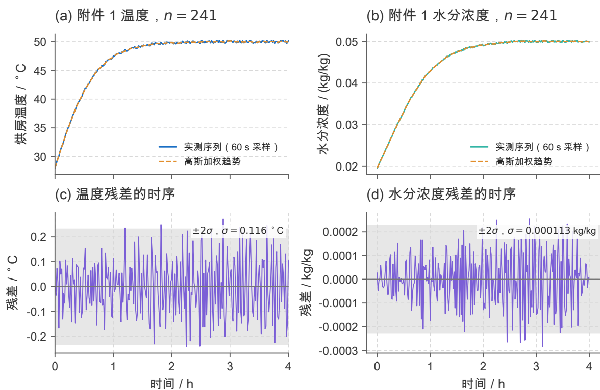
图2 附件1实测序列与噪声诊断 ( n = 241 , 间隔 60 s)。(a)(b) 实测序列 (实线) 与高斯加权局部二次趋势 (虚线, 窗口 15 点、无相位滞后); (c)(d) 相对趋势的残差, 灰带为 \pm 2\sigma 。残差呈高频交替型, 最大幅值仅约 2.3\sigma , 无异常点、无缺失。
