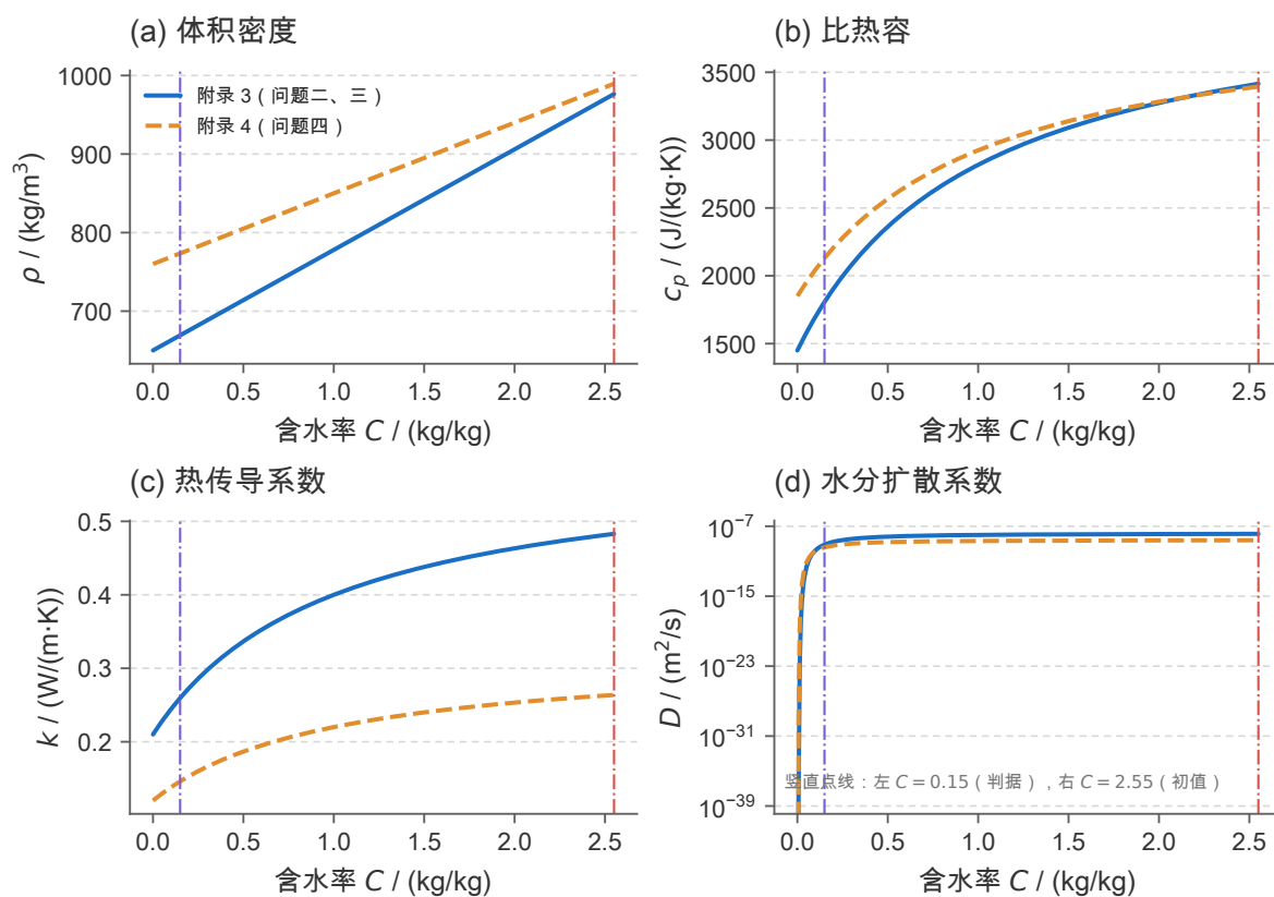
图 8 附录 3、附录 4 的物性随含水率的变化（竖直点线标出初值 C_0 = 2.55 与判据 C = 0.15 ）。(a) 体积密度 \rho 近似线性上升；(b) 比热容 c_p 、(c) 热传导系数 k 均为 C/(C+1) 的线性函数，在 C \rightarrow \infty 时趋于水的物性；(d) 水分扩散系数 D 从初值到判据值下降约 7 倍（若按同一温度比较则约 17 倍），这正是干燥后期“极慢”的根本原因—— e^{-0.45/C} 一项在低含水率下急剧衰减， C 再降到 0.05 时相对 0.15 又跌去 98%（见第 10.4 节的干壳分析）。四张子图共用同一横轴范围，便于横向比较。
