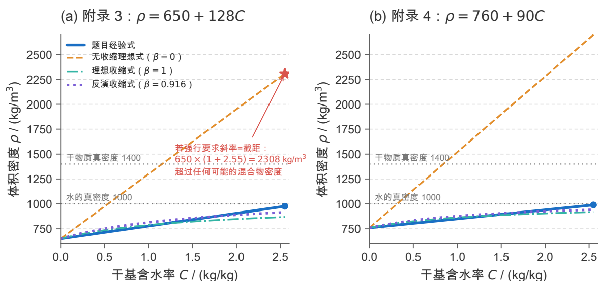
图 4 不同收缩假设下的 \rho-C 关系。实线为题目给定的经验式，其余三条为收缩模型式 (6) 在 \beta = 0 (无收缩)、 \beta = 1 (理想收缩) 与反演值 \beta_{\text{LSQ}} 下的曲线；水平点线为水的真密度 1000 \text{ kg/m}^3 与干物质真密度 1400 \text{ kg/m}^3 。(a) 中的五角星标出“若强行要求斜率等于截距”时的后果： C_0 = 2.55 处将得到 \rho = 2307.5 \text{ kg/m}^3 ，超过水与干物质真密度所能构成的任何混合物密度，物理上不可能。真正不可能的是“斜率等于截距”这一要求本身，而题面经验式与 \beta \approx 0.9 的收缩模型高度吻合。
