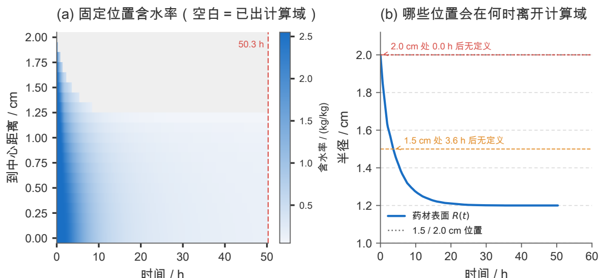
图 12 问题四的含水率时空场与计算域变化。(a) 在固定物理位置上给出的含水率云图：随着半径收缩，1.5 cm 与 2.0 cm 两列先后失去定义（图中灰色区域），这正是表 16 中以“——”表示的原因，也是题面模板允许留空的依据；(b) 药材表面 R(t) 与两条水平参考线的交点标出了“哪些位置会在何时离开计算域”：2.0 cm 处除初始时刻外均已越界，1.5 cm 处自 3.6 h 起无定义（1.0 cm 处始终在药材内部）。
