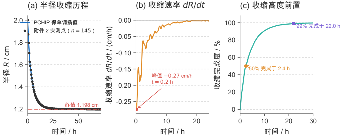
图3 附件2的半径序列与收缩特征 ( n = 145 , 间隔 1800 s)。(a) 实测点与 PCHIP 保单调插值曲线, 半径由 2.000 cm 单调收缩至 1.198 cm; (b) 由 PCHIP 解析导数给出的收缩速率 \dot{R}(t) , 峰值 -0.27 cm/h 出现在最初半小时内, 说明收缩在干燥初期最剧烈; (c) 收缩完成度: 50% 的收缩在 2.5 h 内完成、99% 在 22.0 h 内完成, 收缩高度前置。用差分而非解析导数会把噪声放大 1/\Delta t 倍而看不出这一结构。
