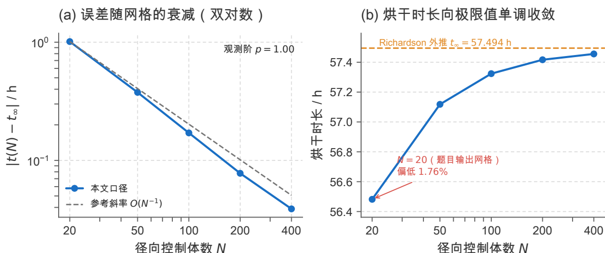
图 13 网格收敛性的定量刻画 (数据同表 17)。(a) 误差 |t(N) - t_\infty| 对网格数 N 的双对数图, 灰色虚线为斜率 -1 的参考线, 实测数据的观测阶为 p = 1.00 , 说明空间格式是一阶收敛 (时间上采用后向 Euler, 空间上采用节点中心有限体积, 一阶是符合预期的); (b) 烘干时长向 Richardson 外推极限 t_\infty = 57.494 h 单调收敛, 题目自带的输出网格 N = 20 偏低 1.76%。两图共同支持”求解网格必须细于输出网格”这一结论。
