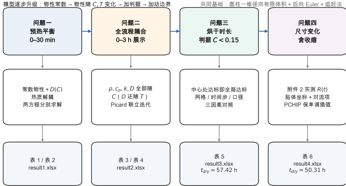
图 1 全文技术路线：四问是同一个模型的四次升级。共同基础是圆柱坐标系下的一维径向耦合传热传质方程、节点中心有限体积、后向 Euler 全隐式推进与追赶法求解；在此基础上依次引入变物性（问题二）→ 两阶段工况与干燥判据（问题三）→ 移动边界（问题四）。四个问题具有一套共同的基础，保证了结论之间的自洽与可比。
