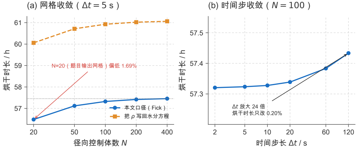
图 14 空间与时间离散的收敛性 (数据同表 17 与表 18)。(a) 固定 \Delta t = 5 \text{ s} , 改变径向控制体数 N : 本文口径与“把 \rho 写回水分方程”的变密度口径给出一对相互平行的收敛曲线, 说明口径差是模型层面的平移, 与网格无关; (b) 固定 N = 100 , 把时间步放大 24 倍, 烘干时长只改变 0.20%, 时间离散误差比空间离散小一个数量级。两图均为确定性计算, 不含统计误差。
