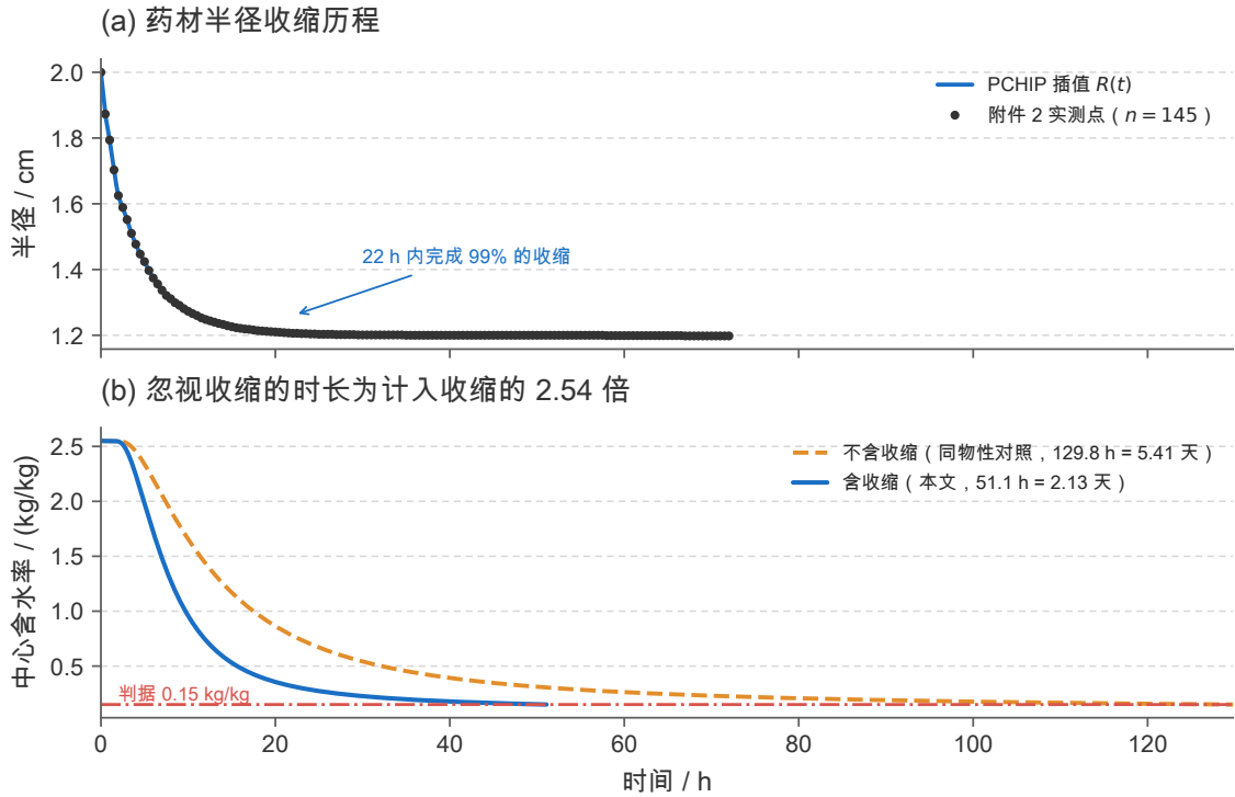
图 2 问题四：收缩历程与烘干时长的对照（附录 4 物性， N = 200 、 \Delta t = 5\text{ s} ）。(a) 附件 2 的实测半径（ n = 145 ，间隔 1800\text{ s} ，实测点以散点示出）与保单调三次 Hermite 插值曲线；插值后 \dot{R} \leq 0 恒成立、无过冲。(b) 中心水分浓度随时间的变化：含收缩时 51.08\text{ h} 达标，固定半径的对照工况需 129.81\text{ h} ，收缩使烘干时长缩短约 61%。两图均为确定性数值结果，不含统计误差。
