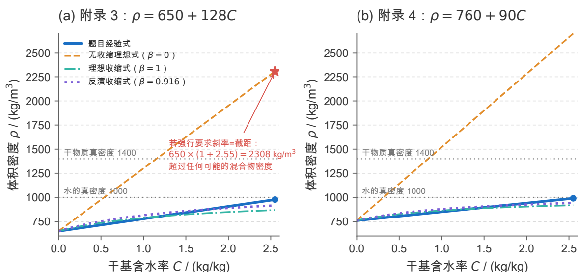
图 3 不同收缩假设下的 \rho-C 关系。实线为题目给定的经验式，其余三条为收缩模型式 (6) 在 \beta = 0 (无收缩)、 \beta = 1 (理想收缩) 与反演值 \beta_{\text{LSQ}} 下的曲线；水平点线为水的真密度 1000 \text{ kg/m}^3 与干物质真密度 1400 \text{ kg/m}^3 。(a) 中的五角星标出“若强行要求斜率等于截距”时的后果： C_0 = 2.55 处将得到 \rho = 2307.5 \text{ kg/m}^3 ，超过水与干物质真密度所能构成的任何混合物密度，物理上不可能。真正不可能的是“斜率等于截距”这一要求本身，而题面经验式与 \beta \approx 0.9 的收缩模型高度吻合。
