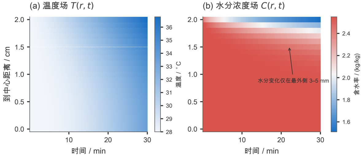
图 5 问题一温度场与水分浓度场的时空演化（节点中心有限体积， N = 400 、 \Delta t = 1 s，图中纵轴为 21 个输出节点）。颜色即数值本身，无色差含义。(a) 热量在 1800 s 内已传遍整个截面， t = 1800 s 时中心 33.58^\circ\text{C} 、表面 36.79^\circ\text{C} ；(b) 水分变化被限制在最外侧约 3 ~ 5 mm 的薄层内，中心含水率在四位小数内始终保持 2.5500 kg/kg。
