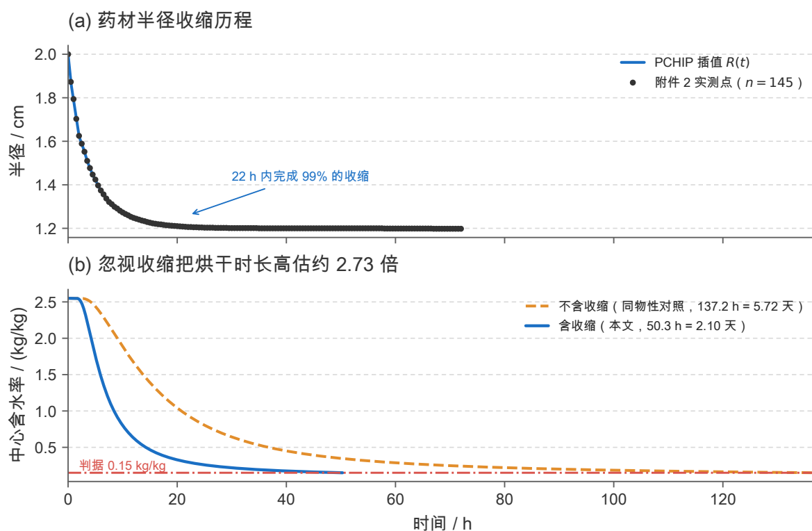
图 10 问题四：收缩历程与烘干时长的对照（附录 4 物性， N = 200 、 \Delta t = 5 s）。(a) 附件 2 的实测半径（ n = 145 ，间隔 1800 s，实测点以散点示出）与保单调三次 Hermite 插值曲线；插值后 \dot{R} \leq 0 恒成立、无过冲。(b) 中心水分浓度随时间的变化：含收缩时 50.31 h 达标，固定半径的对照工况需 137.20 h，收缩使烘干时长缩短约 63%。两图均为确定性数值结果，不含统计误差。
