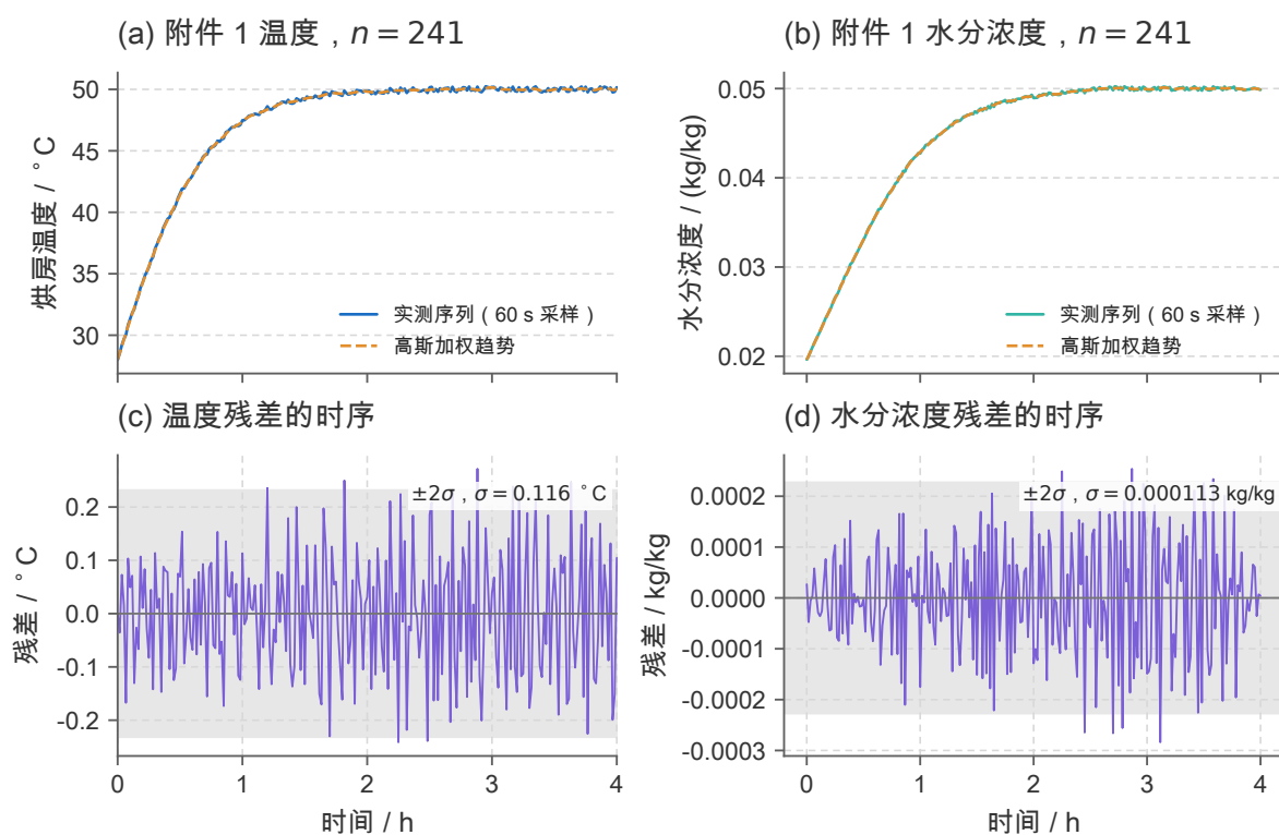
图 1 附件 1 实测序列与噪声诊断 ( n = 241 , 间隔 60 s)。 (a)(b) 实测序列 (实线) 与高斯加权局部二次趋势 (虚线, 窗口 15 点、无相位滞后); (c)(d) 相对趋势的残差, 灰带为 \pm 2\sigma 。残差呈高频交替型, 最大幅值仅约 2.3\sigma , 无异常点、无缺失。
