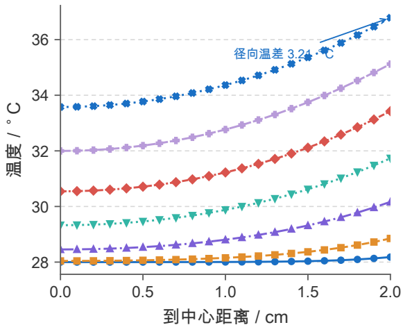
(a) 温度剖面
