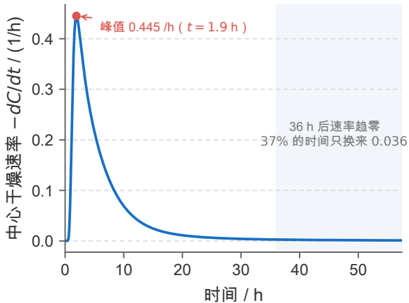
(a) 干燥速率的时间历程
