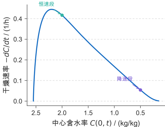
(b) 干燥速率曲线 (对含水率)
