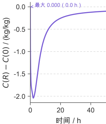
(b) 内外含水率之差
