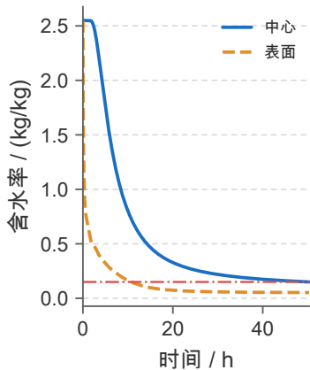
(a) 中心与表面历程
