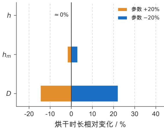
(a) 三类参数的灵敏度
