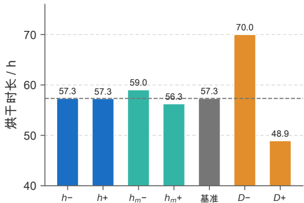
(b) 绝对烘干时长
