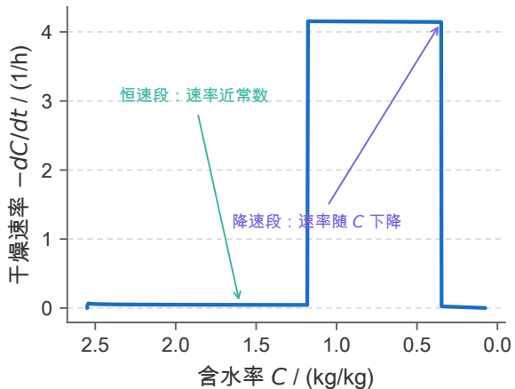
(b) 干燥速率曲线 (示意)
