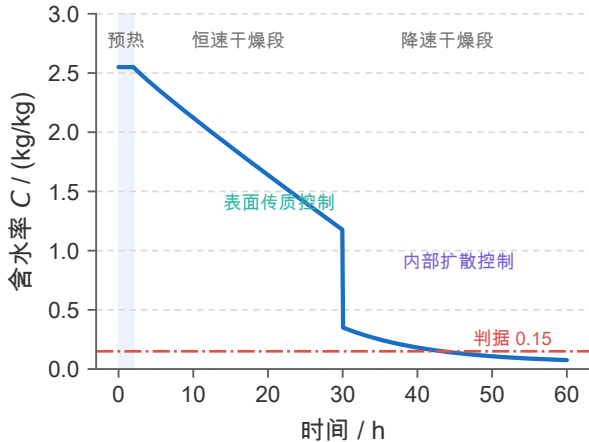
(a) 含水率历程的三段结构 (示意)
