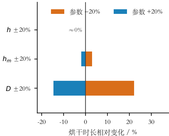
(a) 关键参数的灵敏度 (基准 57.32 h)
