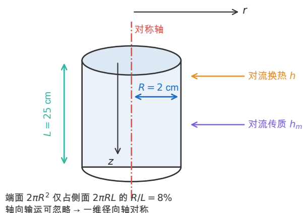
图 10 圆柱形药材的几何、柱坐标与一维径向简化。(a) 几何与坐标架：药材长 L = 25\text{ cm} 、半径 R = 2\text{ cm} ，取柱坐标 (r, z) ， r 为到中心轴的距离、 z 为轴向；侧面同时发生对流换热 ( h ) 与对流传质 ( h_m )，端面面积 2\pi R^2 仅占侧面积 2\pi RL 的 R/L = 8\% ，故轴向输运可忽略。(b) 横截面上的简化：由轴对称性，场量与周向角无关，问题退化为一维径向问题 T(r, t) 、 C(r, t) ；中心 r = 0 为对称边界 ( \partial_r T = \partial_r C = 0 )，表面 r = R 为第三类边界；蓝色环状区域即后文有限体积离散所用的控制体 2\pi r dr dz 。
