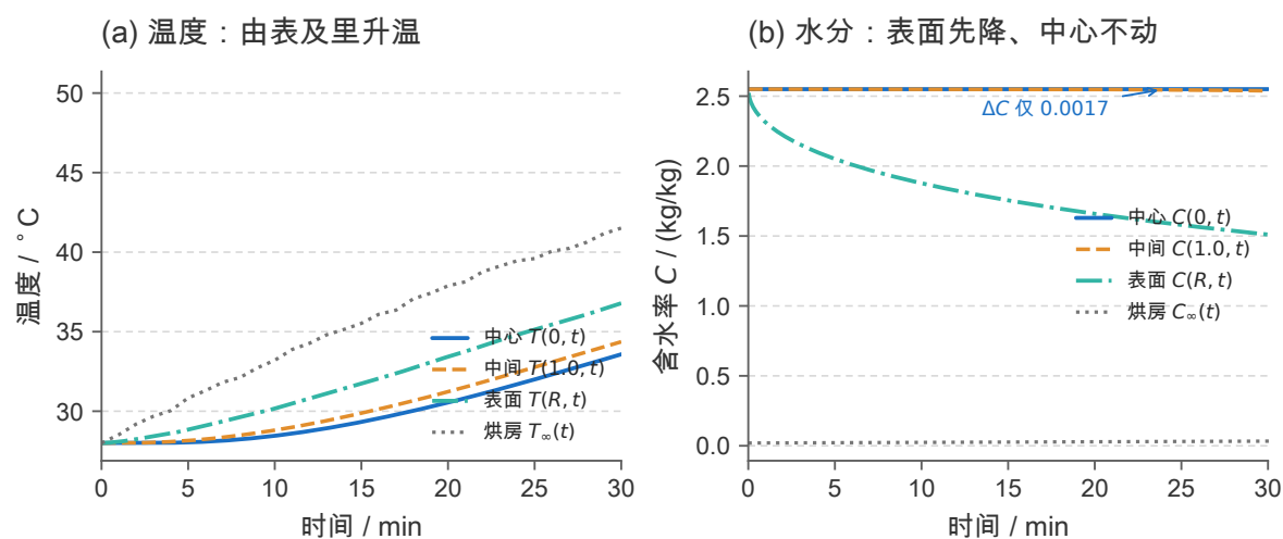
图 17 问题一中心 / 中间 / 表面与烘房状态的时间历程。(a) 温度：表面升温最快、中心最慢，30 min 内中心由 28.00 °C 升到 33.58 °C、表面升到 36.79 °C；(b) 水分浓度：表面由 2.5500 降到 1.5103，而中心在 30 min 内仅变化 0.0017。”温度全场重分布、水分只动表层”的对比是预热平衡阶段最本质的物理特征。
