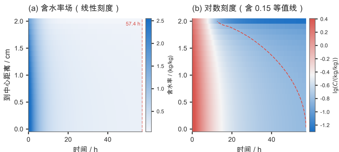
图 32 问题三全过程的含水率时空云图。(a) 线性色标: 低含水率区间的层次被压得很扁; (b) 对数色标并叠加 C = 0.15 等值线 (红虚线), 可以清楚看到干燥前沿由表面向中心推进, 等值线在 57.4 h 才扫过中心轴。之所以并排给出两种色标, 是因为判据附近的数值区间很窄, 只有对数刻度才看得出层次; 两图均附 colorbar 并标出单位。
