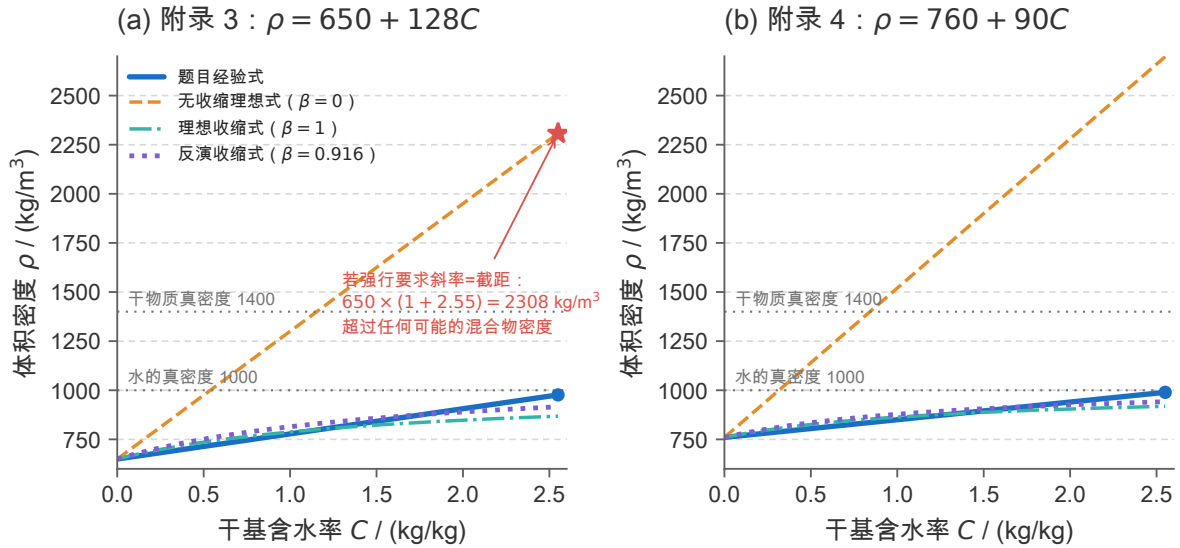
图 6 不同收缩假设下的 \rho - C 关系。实线为题目给定的经验式，其余三条为收缩模型式 (6) 在 \beta = 0 (无收缩)、 \beta = 1 (理想收缩) 与反演值 \beta_{\text{LSQ}} 下的曲线。水平点线为水的真密度 1000 \text{ kg/m}^3 与干物质真密度 1400 \text{ kg/m}^3 。(a) 中的五角星标出“若强行要求斜率等于截距”时的后果：在 C_0 = 2.55 处将得到 \rho = 650 \times 3.55 = 2307.5 \text{ kg/m}^3 ，超过水与干物质真密度所能构成的任何混合物密度，物理上不可能。真正不可能的恰恰是“斜率等于截距”这一要求本身，而题目经验式与 \beta \approx 0.9 的收缩模型高度吻合。本图为解析计算，不含数值误差。
