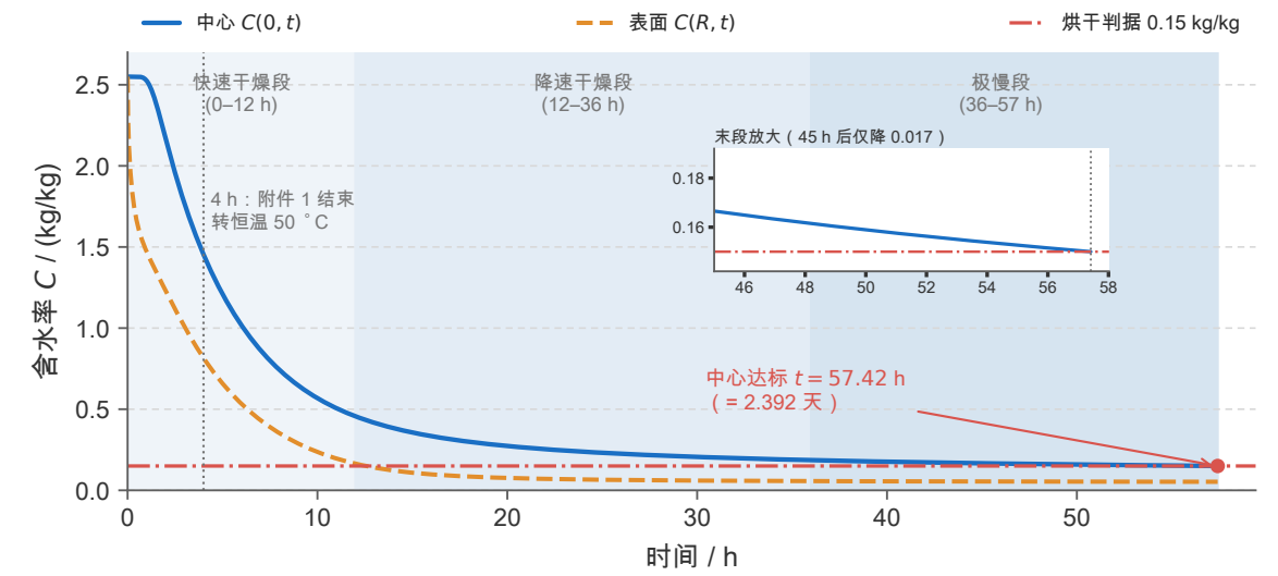
图 30 问题三干燥曲线：中心与表面水分浓度随时间的变化（ N = 200 、 \Delta t = 5\text{ s} ，判据为各点 C < 0.15\text{ kg/kg} ）。红色点划线为烘干判据 0.15 kg/kg，阴影区依次为快速干燥段（0–12 h）、降速干燥段（12–36 h）与极慢干燥段（36–57.42 h）；后者耗时 21 h 却只换来 0.036 kg/kg 的下降。表面自 14.2 h 起即已达标（占全程 23%），全程由中心决定。竖向点线标出 4 h 处的阶段转换（附件 1 结束、转入恒温 50 °C 工况）；右上角插图把”最后 12 h 只降 0.017”这一反直觉结论直接呈现出来。
