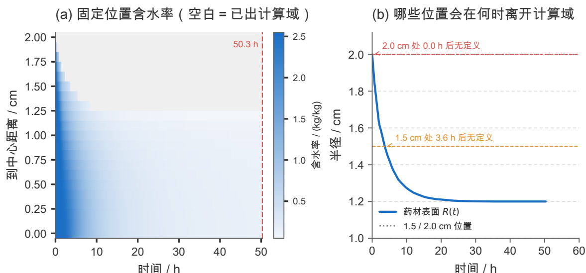
图 39 问题四的含水率时空场与计算域变化。(a) 在固定物理位置上给出的含水率云图：随着半径收缩，1.5 cm 与 2.0 cm 两列先后失去定义（图中灰色区域），这正是表 22 中以“——”表示的原因，也是题面模板允许留空的依据；(b) 药材表面 R(t) 与两条水平参考线的交点标出了“哪些位置会在何时离开计算域”：2.0 cm 处除初始时刻外均已越界，1.5 cm 处自 3.6 h 起无定义（1.0 cm 处始终在药材内部）。
