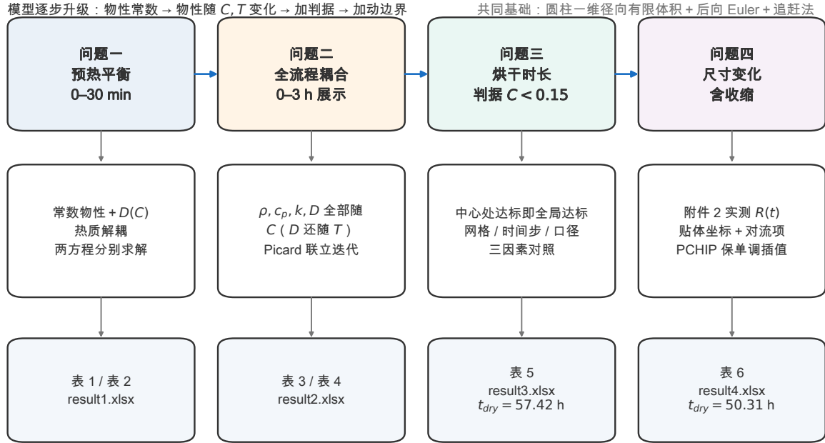
图 1 全文技术路线：四问不是四个模型，而是同一个模型的四次升级。共同基础是圆柱坐标系下的一维径向耦合传热传质方程、节点中心有限体积、后向 Euler 全隐式推进与追赶法求解；在此基础上依次引入变物性（问题二）→ 两阶段工况与干燥判据（问题三）→ 移动边界（问题四）。四个问题共用一套数值格式与同一份程序，保证了结论之间的自洽与可比。
