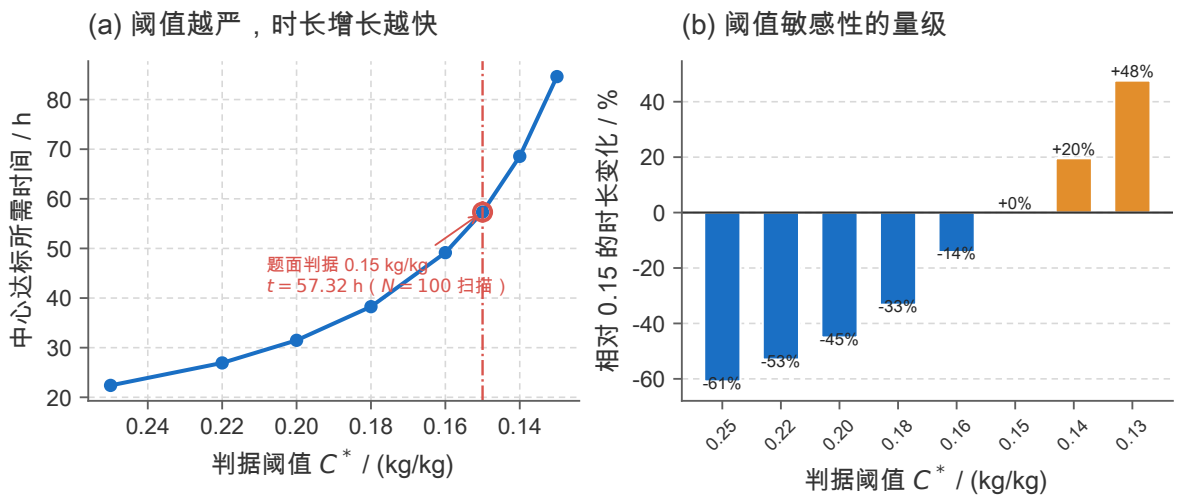
图 34 烘干判据阈值的敏感性 ( N = 100 、 \Delta t = 5 s 扫描)。(a) 中心达标所需时间随阈值的变化：阈值越严，所需时间增长越快，曲线在 C^* 低于 0.16 之后明显变陡；对应的烘干时长为 0.20 \rightarrow 31.5 h 、 0.18 \rightarrow 38.3 h 、 0.16 \rightarrow 49.2 h 、 0.15 \rightarrow 57.3 h 、 0.13 \rightarrow 84.6 h ；(b) 相对题面判据 0.15 的时长变化率：把阈值放宽到 0.20 可省 45% 的时间，放宽到 0.25 可省 61%；而收紧到 0.13 则要多耗 48%。该图给出的是工艺建议的直接依据——在满足品质要求的前提下，判据每放宽 0.01 kg/kg 都能带来可观的时间与能耗收益，且这一结论比单点结果更能体现模型的稳健性。
