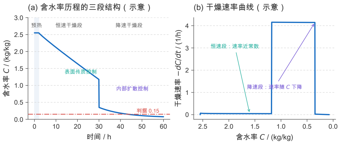
图 29 干燥三阶段的示意（用于说明概念，不是计算结果）。(a) 含水率历程按”预热平衡 → 恒速干燥 → 降速干燥”三段划分，红色点划线为 0.15 kg/kg 判据；(b) 对应的干燥速率曲线：恒速段的速率近似常数，降速段的速率随含水率单调下降。本文的实际结果（图 33）中看不到恒速段平台，原因是题给的 D = 2.4 \times 10^{-3} e^{-0.45/C} e^{-3850/T} 使扩散系数随含水率指数衰减，表面传质从未成为限制环节——这正是本题区别于经典恒速干燥的一个特点。
