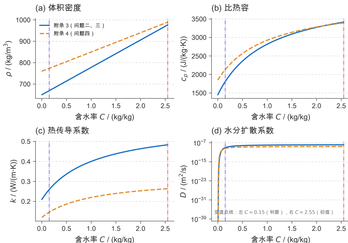
图24 附录3、附录4的物性随含水率的变化（竖直线标出初值 C_0 = 2.55 与判据 C = 0.15 ）。(a) 体积密度 \rho 近似线性上升；(b) 比热容 c_p 、(c) 热传导系数 k 均为 C/(C+1) 的线性函数，在 C \rightarrow \infty 时趋于水的物性；(d) 水分扩散系数 D 从初值到判据值下降约两个数量级，这正是干燥后期“极慢”的根本原因—— e^{-0.45/C} 一项在低含水率下急剧衰减。四张子图共用同一横轴范围，便于横向比较。
