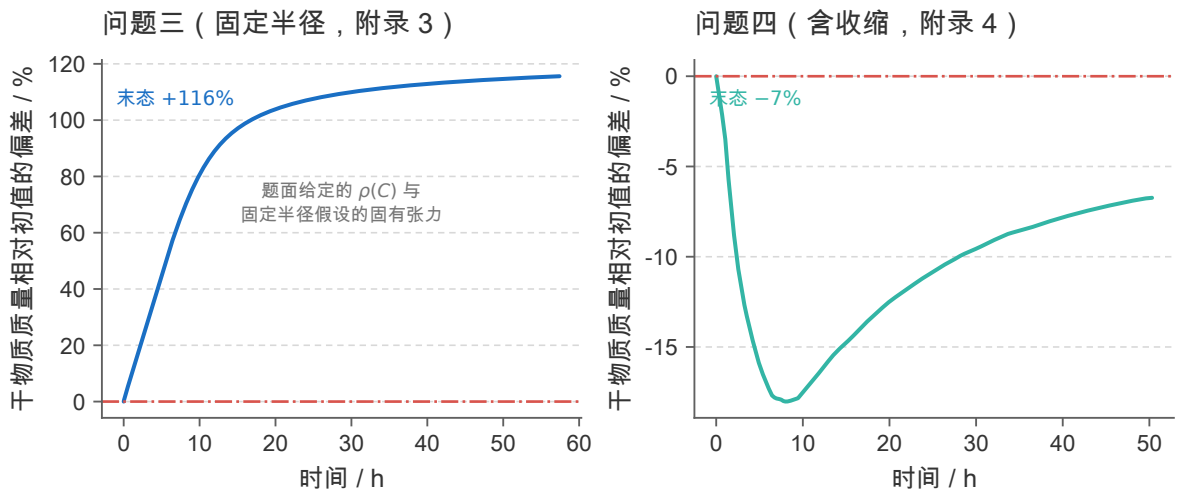
图 26 干物质质量的守恒性检验：按式 (40) 用已求得的 C(r,t) 与附件 2 的实测 R(t) 反算单位长度的干料质量，并以其初值为基准归一。左：问题三（固定半径、附录 3）的偏差单调增大到 +116%；右：问题四（含收缩、附录 4）在 2 h 滑动平均后稳定在 −7% 附近（未平滑的原始曲线因半径越过 0.1 cm 网格线而带采样锯齿）。左图的系统性增长即“密度经验式隐含收缩”与“固定半径假设”之间的矛盾在两问中的体现，与图 9(b) 半径对照给出的 −19.5% 差异互为佐证。
