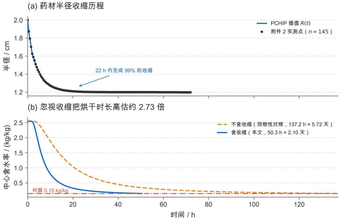
图 38 问题四：收缩历程与烘干时长的对照（附录 4 物性， N = 200 、 \Delta t = 5 s）。(a) 附件 2 的实测半径（ n = 145 ，间隔 1800 s，实测点以散点示出）与保单调三次 Hermite 插值曲线；插值后 \dot{R} \leq 0 恒成立、无过冲。(b) 中心水分浓度随时间的变化：含收缩时 50.31 h 达标，固定半径的对照工况需 137.20 h，收缩使烘干时长缩短约 63%。两图均为确定性数值结果，不含统计误差。
