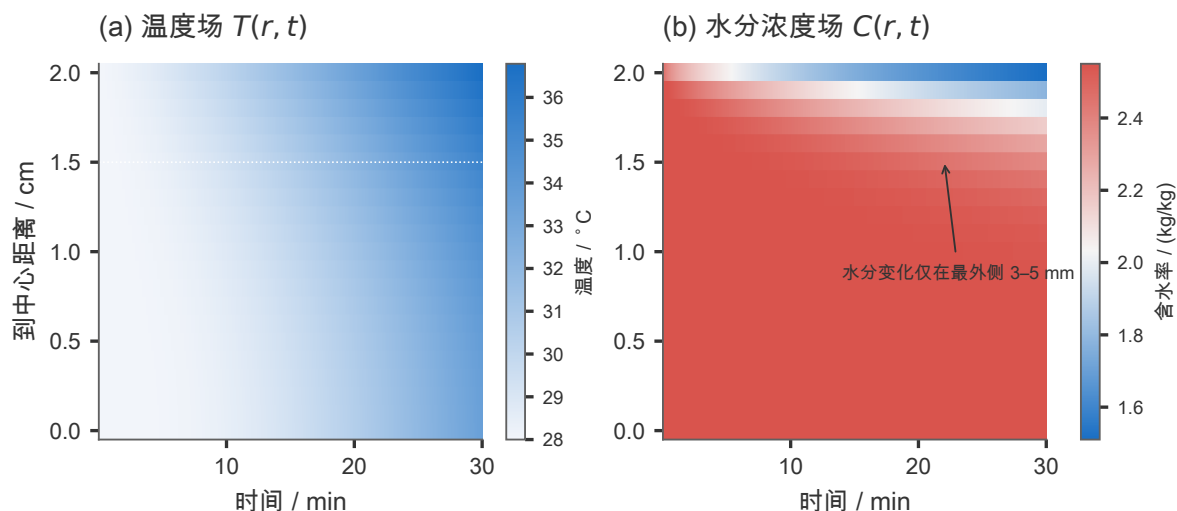
图 15 问题一温度场与水分浓度场的时空演化（节点中心有限体积， N = 400 、 \Delta t = 1 s，图中纵轴为 21 个输出节点）。颜色即数值本身，无色差含义。(a) 热量在 1800 s 内已传遍整个截面， t = 1800 s 时中心 33.58^\circ\text{C} 、表面 36.79^\circ\text{C} ；(b) 水分变化被限制在最外侧约 3 ~ 5 mm 的薄层内，中心含水率在四位小数内始终保持 2.5500 kg/kg。
