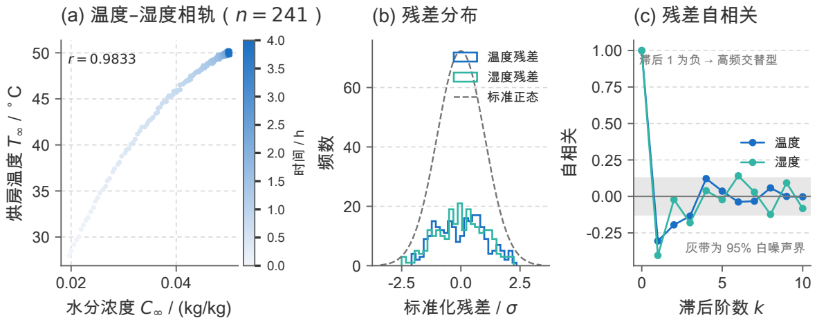
图3 附件1的数据质量诊断。(a) 温度-湿度相轨，颜色为时间，两者高度同向（ r = 0.983 ），说明烘房升温与排湿是同一个工况推进过程；(b) 两条序列标准化残差的分布与标准正态对照，均近似对称、无重尾；(c) 残差自相关函数，滞后1阶为负且落在95%白噪声带之外，是高频交替型噪声（传感器噪声或控温往复调节）而非真实物理起伏的直接证据——这正是下文“不对附件1作平滑”的主要依据之一。
