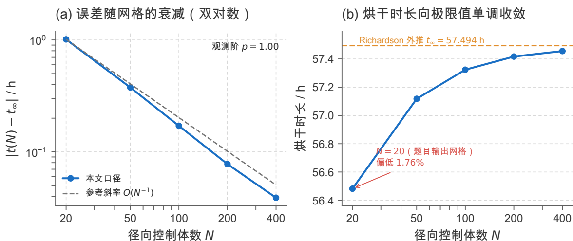
图 35 网格收敛性的定量刻画 (数据同表 17)。(a) 误差 |t(N) - t_\infty| 对网格数 N 的双对数图, 灰色虚线为斜率 -1 的参考线, 实测数据的观测阶为 p = 1.00 , 说明空间格式是一阶收敛 (时间上采用后向 Euler, 空间上采用节点中心有限体积, 一阶是符合预期的); (b) 烘干时长向 Richardson 外推极限 t_\infty = 57.494 h 单调收敛, 题目自带的输出网格 N = 20 偏低 1.76%。两图共同支持”求解网格必须细于输出网格”这一结论。
