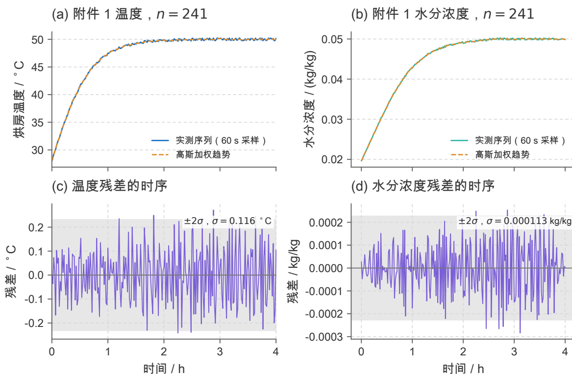
图 2 附件 1 实测序列与噪声诊断 ( n = 241 , 采样间隔 60 s)。 (a)(b) 烘房温度与水分浓度的实测序列 (实线) 与高斯加权局部二次趋势 (虚线, 窗口 15 点、无相位滞后); (c)(d) 两条序列相对各自趋势的残差, 灰色带为 \pm 2\sigma , 温度残差 \sigma = 0.116^{\circ}\text{C} 、水分浓度残差 \sigma = 1.1 \times 10^{-4} \text{ kg/kg} 。残差呈高频交替型 (滞后 1 自相关为负), 最大幅值仅约 2.3\sigma , 无异常点、无缺失。
