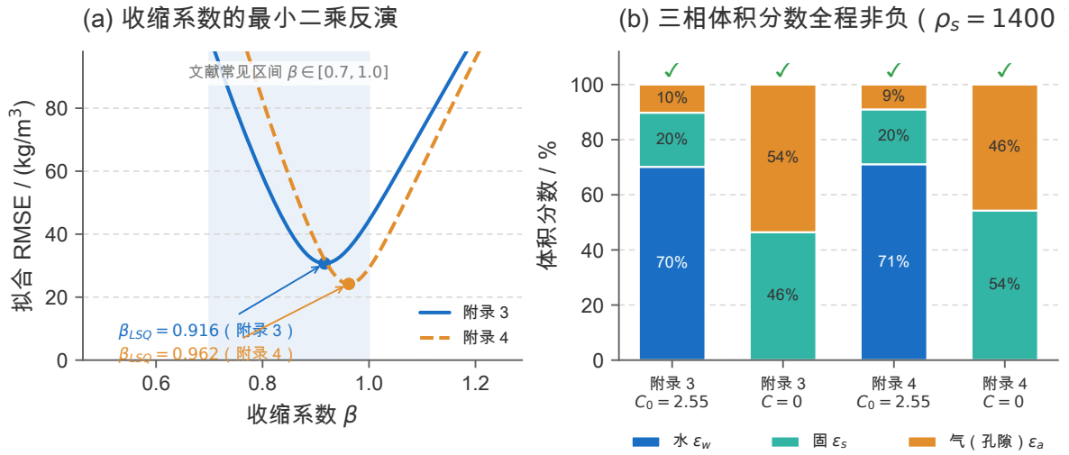
图 8 (a) 收缩系数的最小二乘反演：横轴为 \beta ，纵轴为双曲式 (6) 对线性式的拟合 RMSE，圆点为最优值；阴影带为文献中果蔬、中药材常见的 \beta \in [0.7, 1.0] 。(b) 三相体积分数（水 / 固 / 气）在初始湿态与完全干燥态的分布，四种情形下三相均非负（通过），孔隙率量级与植物材料相符。
