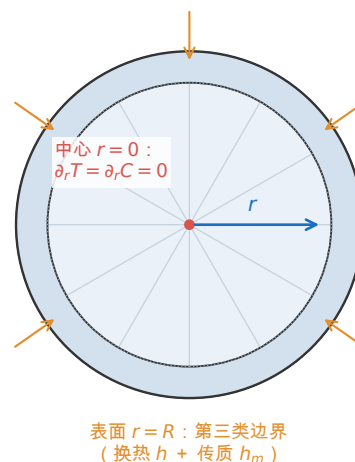
图 10 圆柱形药材的几何、柱坐标与一维径向简化。(a) 几何与坐标架：药材长 L = 25\text{ cm} 、半径 R = 2\text{ cm} ，取柱坐标 (r, z) ， r 为到中心轴的距离、 z 为轴向；侧面同时发生对流换热 ( h ) 与对流传质 ( h_m )，端面面积 2\pi R^2 仅占侧面积 2\pi RL 的 R/L = 8\% ，故轴向输运可忽略。(b) 横截面上的简化：由轴对称性，场量与周向角无关，问题退化为一维径向问题 T(r, t) 、 C(r, t) ；中心 r = 0 为对称边界 ( \partial_r T = \partial_r C = 0 )，表面 r = R 为第三类边界；蓝色环状区域即后文有限体积离散所用的控制体 2\pi r dr dz 。
