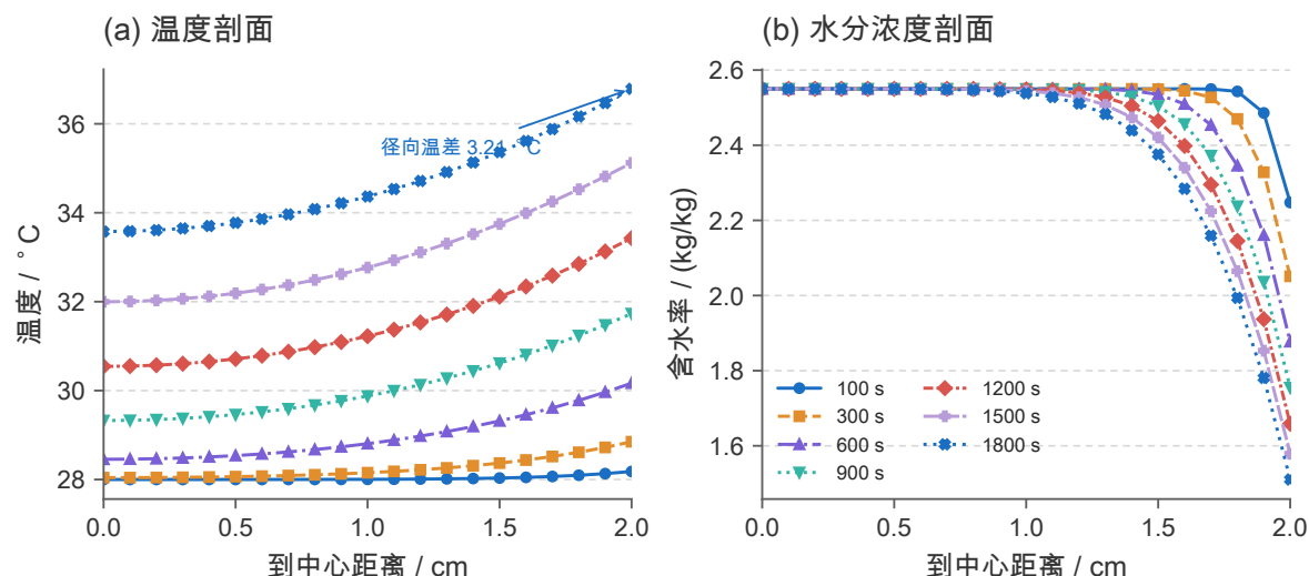
图 16 问题一各报数时刻的径向剖面（即表 8、9 的 100–1800 s 七行）。(a) 温度：整条剖面随时间整体抬升，且始终“外高内低”；(b) 水分浓度：0 ~ 1.0 cm 的曲线几乎完全重合，只有 1.5 cm 与 2.0 cm 处明显下降，直观印证“水分只动了最外侧 3 ~ 5 mm”。两图均采用线型 + 标记的双重编码，黑白打印时仍可分辨各时刻。
