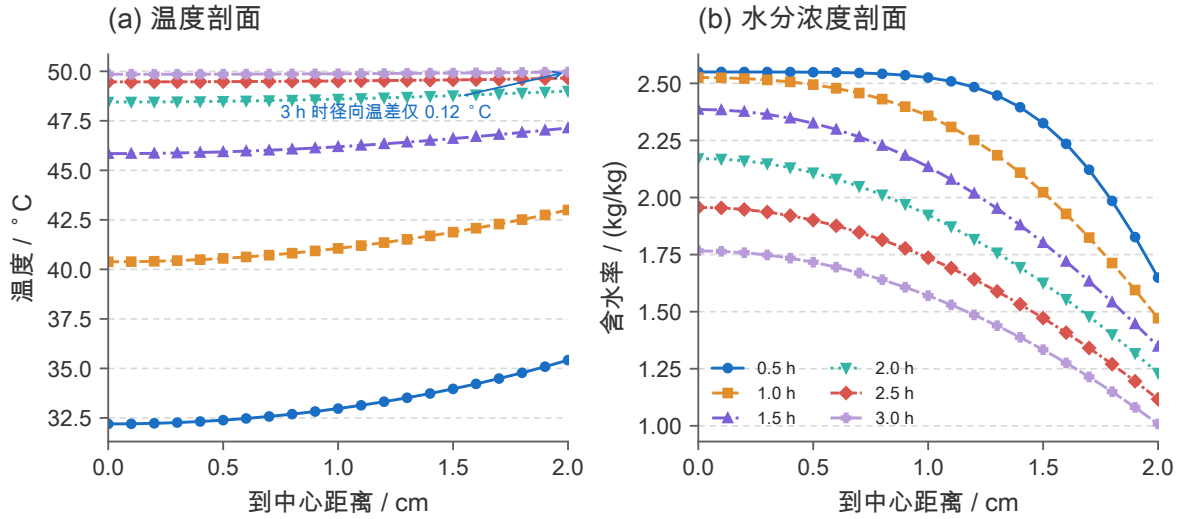
图 21 问题二 3 h 内温度与水分浓度的径向剖面（附录 3 变物性耦合模型， N = 200 、 \Delta t = 5 s，曲线取自 0 ~ 2.0 cm 等距 21 个输出节点）。6 条曲线分别对应 0.5、1.0、1.5、2.0、2.5、3.0 h，以线型与标记作冗余编码以适配色觉异常读者。(a) 2.5 h 后温度趋于均匀，3 h 时径向温差仅 0.12 °C；(b) 含水率始终保留由内向外的正梯度，说明过程由内部扩散控制。
