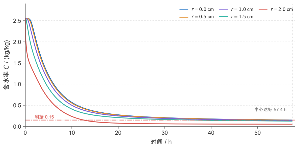
图 31 问题三各径向位置的含水率历程族 ( r = 0, 0.5, 1.0, 1.5, 2.0 cm)。五条曲线在 10 h 之前彼此分离, 之后逐渐收拢并长期并行下降; 最外层的 2.0 cm 曲线最早穿越判据 (约 14.2 h), 中心 0 cm 最晚 (57.42 h)。判据的控制点始终是中心, 这正是把“各处达标”等价为 C(0, t) < 0.15 的图形依据。
