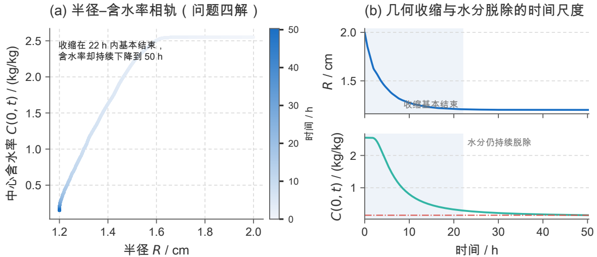
图 5 半径与含水率的对应关系（数据取自问题四的解）。(a) 以时间为颜色的半径-含水率相轨：轨迹在相平面上先快速左移（半径迅速减小）、再长时间下移（含水率继续脱除）；(b) 把两个量纲不同的量拆成上下两个共享时间轴的子图（不用双纵轴）：收缩在 22 h 内基本结束，而含水率的缓慢下降持续到 50 h 之后，两者相差一个量级。因此不能假定 R 与 C 同步，本文直接采用实测 R(t) 。
