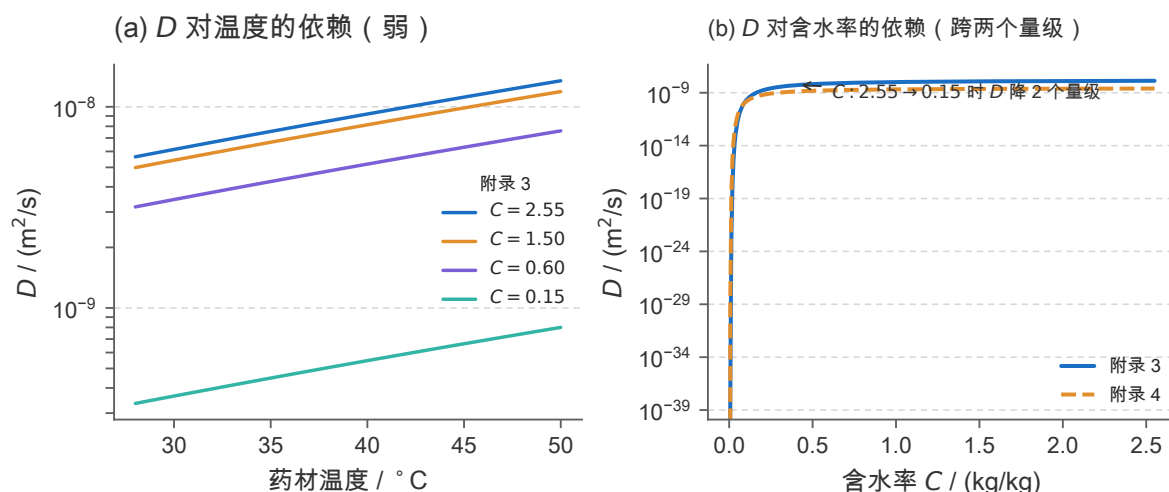
图25 水分扩散系数 D 的两个依赖关系。(a) 对温度的依赖：在 28 \rightarrow 50^\circ\text{C} 区间内各条曲线都是缓升的指数函数， \exp(-3850/T) 使 D 整段增大约 2.39 倍 (+139%)，与含水率带来的两个数量级相比是次要因素；(b) 对含水率的依赖： C 由 2.55 降到 0.15 时 D 下降两个量级，是主控因素。注意两图的纵轴均为对数轴，且附录3、4的 D 相差约两个数量级，口径不可混用。
