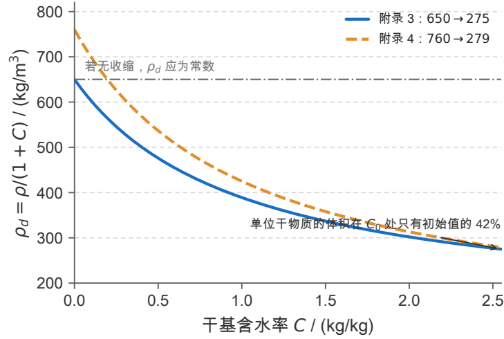
图 7 由题目经验式反算的表观干物质密度 \rho_d = \rho / (1 + C) 。两条曲线都随含水率单调下降，说明 \rho_d 不是常数；灰色点线给出“若无收缩则 \rho_d 应为常数”的参照。
