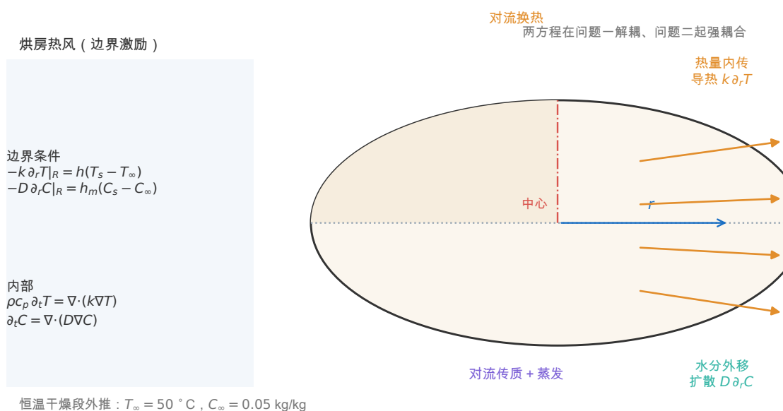
图 11 预热平衡阶段的物理图像与两条传输通道。烘房空气状态 T_\infty(t) 、 C_\infty(t) 是边界激励；药材内部温度由导热 k \partial_r T 向内传递，水分由扩散 D \partial_r C 向外迁移，两者在表面通过第三类边界与空气交换。左侧给出内部方程与表面边界条件，右上角点明本文的结构性结论：两个方程在问题一解耦、自问题二起强耦合。
