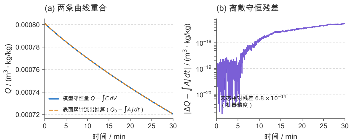
图 19 问题一的离散守恒性检验。(a) 模型守恒量 Q = \int C dV 的下降曲线与由表面累计通量 \int A_j dt 反推的曲线完全重合；(b) 两者之差（对数纵轴）始终处于机器精度量级，1800 s 末态的相对残差为 6.8 \times 10^{-14} 。需要强调守恒量应是 \int C dV 而不是 \int \rho_d C dV ——在本文采用的经典 Fick 口径下密度已被约去。
