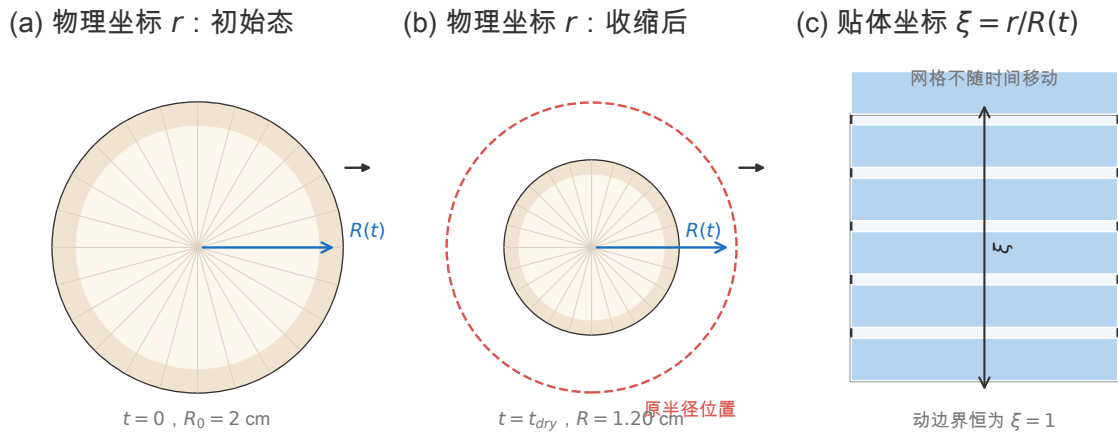
图 37 贴体坐标变换把动边界化为固定区域。(a) 物理坐标下 t = 0 的初始态，网格均匀铺在 r \in [0, R_0] 上；(b) 物理坐标下收缩后的状态，半径缩到 1.20 cm，若仍用固定物理网格，最外侧节点会落到药材之外；(c) 贴体坐标 \xi = r/R(t) 下动边界恒为 \xi = 1 ，网格不随时间移动，代价是方程中多出一个 \xi \dot{R} \partial C / \partial \xi 的对流项。这正是问题四与前三问在数值上的唯一结构性差别。
