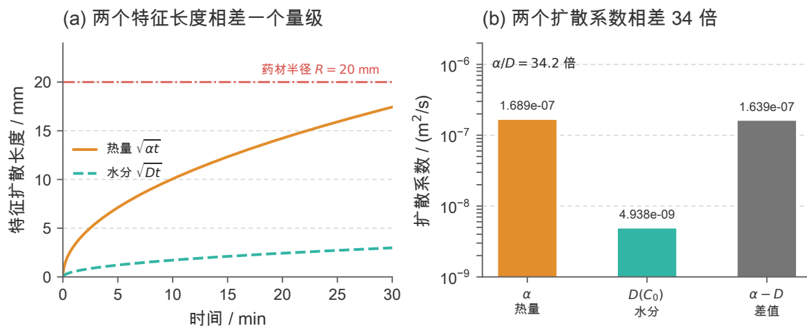
图 18 特征扩散长度与扩散系数的量级对比。(a) 热量的特征扩散长度 \sqrt{\alpha t} 与水分 \sqrt{D t} 随时间的变化：1800 s 时前者达 17.4 mm、已接近半径 R = 20 \text{ mm} ，后者仅 2.98 mm；(b) 两个扩散系数 \alpha = 1.689 \times 10^{-7} 与 D(C_0) = 4.938 \times 10^{-9} \text{ m}^2/\text{s} 相差 34.2 倍。两个数即可解释“温度全场重分布、水分只动最外 3 ~ 5 mm”，也说明表面传质阻力不是限制环节。
