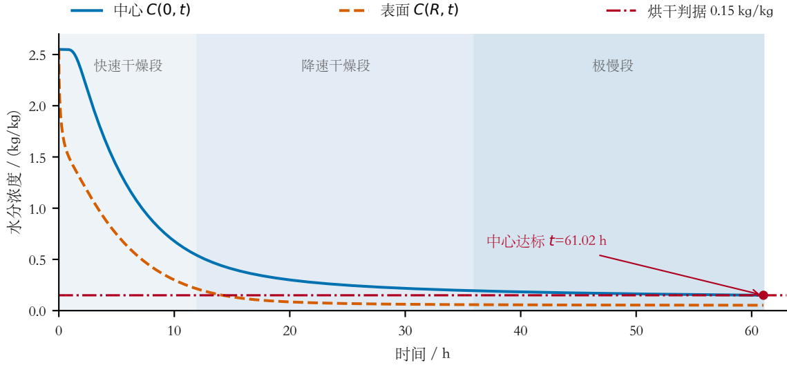
图 6 问题三干燥曲线：中心与表面水分浓度随时间的变化 ( N = 200 、 \Delta t = 5 \text{ s} ，判据为各点 C < 0.15 \text{ kg/kg} )。红色点划线为烘干判据 0.15 \text{ kg/kg} ，阴影区依次为快速干燥段 (0–12 h)、降速干燥段 (12–36 h) 与极慢干燥段 (36–61.02 h)；后者耗时 25 h 却只换来 0.044 \text{ kg/kg} 的下降。表面自 14.2 h 起即已达标（占全程 23%），全程由中心决定。
