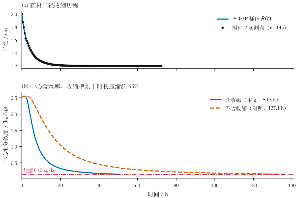
图 7 问题四：收缩历程与烘干时长的对照（附录 4 物性， N = 200 、 \Delta t = 5\text{ s} ）。(a) 附件 2 的实测半径（ n = 145 ，间隔 1800 s，实测点以散点示出）与保单调三次 Hermite 插值曲线；插值后 \dot{R} \leq 0 恒成立、无过冲。(b) 中心水分浓度随时间的变化：含收缩时 50.31 h 达标，固定半径的对照工况需 137.10 h，收缩使烘干时长缩短约 63%。两图均为确定性数值结果，不含统计误差。
