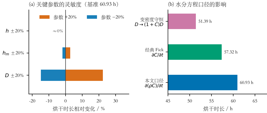
图 5 (a) 关键参数 \pm 20\% 扰动对问题三烘干时长的影响（基准 60.93 h， N = 100 、 \Delta t = 5 s，即表 14 与表 15 中的同一组设定）； h 的条形几乎为零宽，故直接标注 \approx 0\% 。(b) 水分方程三种口径给出的烘干时长，误差来源为方程口径而非数值误差。两图均为确定性计算结果，不含统计误差，故不设误差棒。
