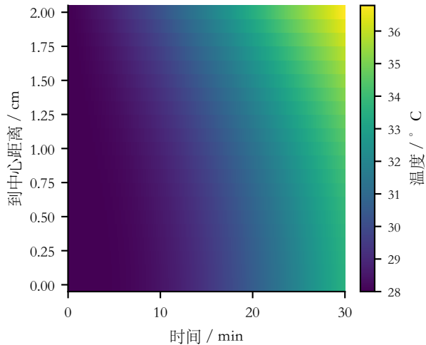
(a) 温度场 T(r, t)
