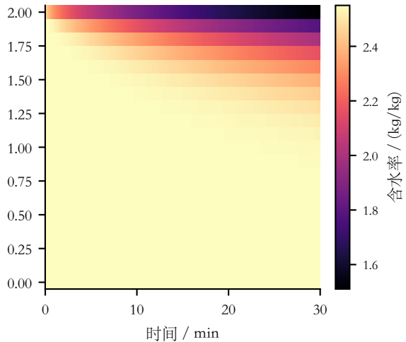
(b) 水分浓度场 C(r, t)
