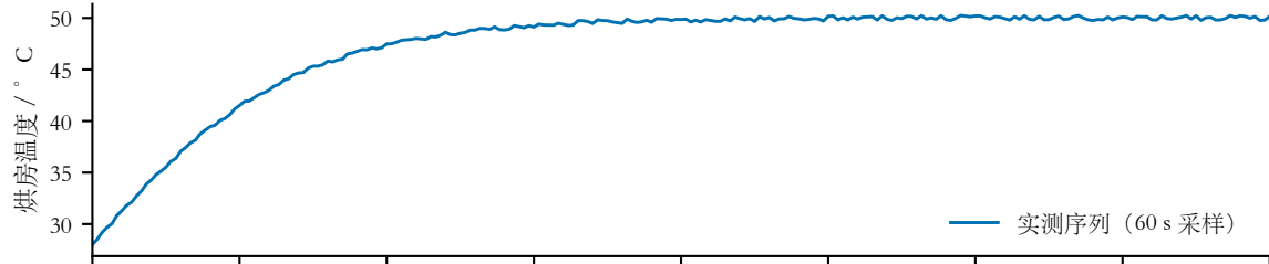
(a) 附件 1 烘房温度
