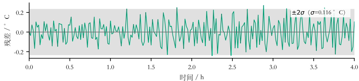
(c) 温度残差：高频交替型噪声，无异常点
