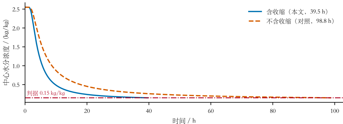
(b) 中心含水率：收缩把烘干时长压缩约 60%
