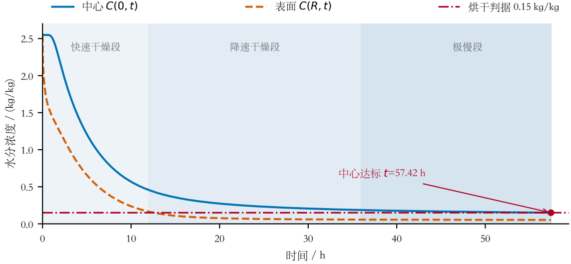
图 6 问题三干燥曲线：中心与表面水分浓度随时间的变化 ( N = 200 、 \Delta t = 5 s, 判据为各点 C < 0.15 kg/kg)。红色点划线为烘干判据 0.15 kg/kg, 阴影区依次为快速干燥段 (0–12 h)、降速干燥段 (12–36 h) 与极慢干燥段 (36–57.42 h); 后者耗时 21 h 却只换来 0.036 kg/kg 的下降。表面自 14.2 h 起即已达标 (占全程 23%), 全程由中心决定。
