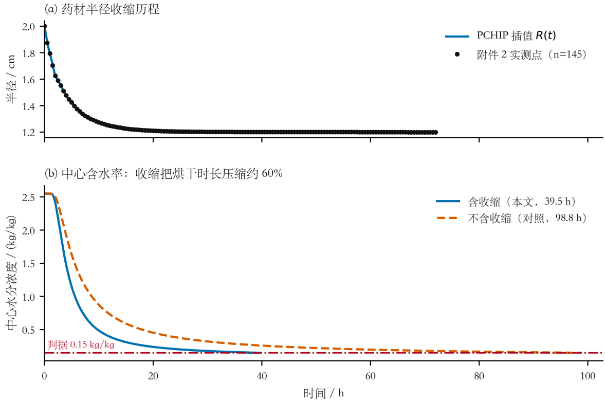
图 7 问题四：收缩历程与烘干时长的对照（附录 4 物性， N = 200 、 \Delta t = 5 s）。(a) 附件 2 的实测半径（ n = 145 ，间隔 1800 s，实测点以散点示出）与保单调三次 Hermite 插值曲线；插值后 R 单调递减、无过冲。(b) 中心水分浓度随时间的变化：含收缩时 39.55 h 达标，固定半径的对照工况需 98.77 h，收缩使烘干时长缩短约 60%。两图均为确定性数值结果，不含统计误差。
