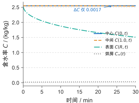
(b) 水分：表面先降、中心不动
