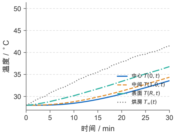
(a) 温度：由表及里升温
