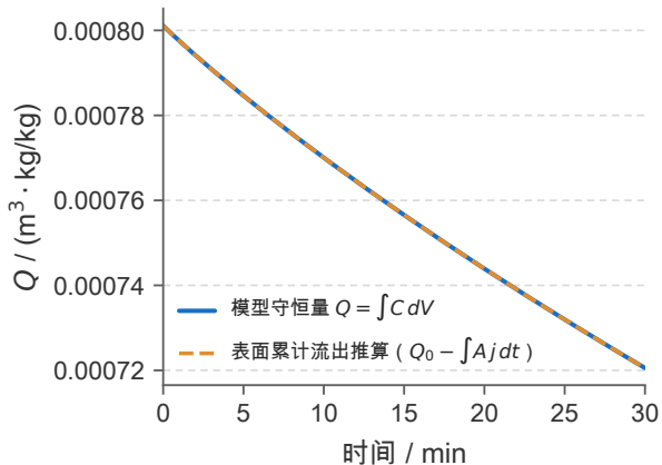
(a) 两条曲线重合
