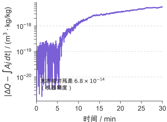
(b) 离散守恒残差
