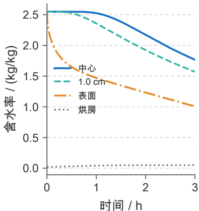
(b) 含水率由表及里依次下降
