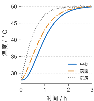
(a) 温度快速趋于均匀
