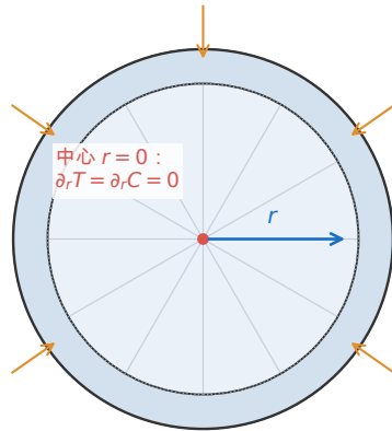
(b) 一维径向简化 (横截面)
