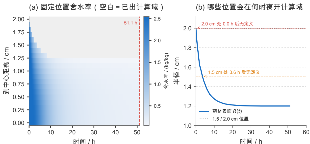
图 7 问题四移动边界下的含水率场：(a) 固定位置含水率，空白表示该位置已随收缩离开计算域；(b) 各半径位置的失效时刻，表面由 2.0 cm 收缩到 1.198 cm。
