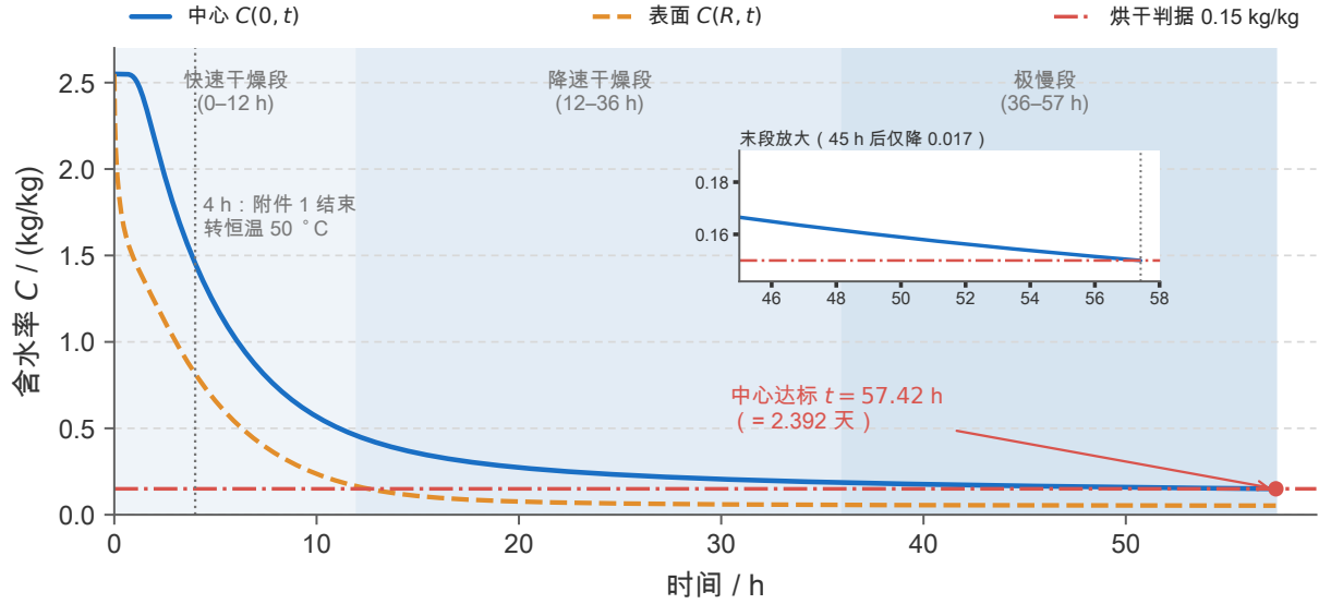
图 5 问题三干燥曲线：中心与表面水分浓度随时间的变化（ N = 200 、 \Delta t = 5 s，判据为各点 C < 0.15 kg/kg），右上角插图为 45 h 之后的放大。
