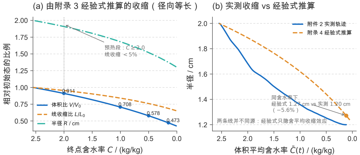
图9 (a) 由附录3经验式推算的几何收缩: 体积比 V/V_0 、线收缩比 L/L_0 与对应半径随终点含水率的变化; C \geq 2.0 时线收缩不足 5% (径向等长口径)。 (b) 由 \rho(C) 反推的 R(C) 与附件2实测 R-C 轨迹的对照 (横轴为体积加权平均含水率 \bar{C} ): 同一含水率下经验式比实测偏大约 5.6%, 外推到绝干则只差 1.1%; 路径上前者与含水率同步、后者高度前置。
