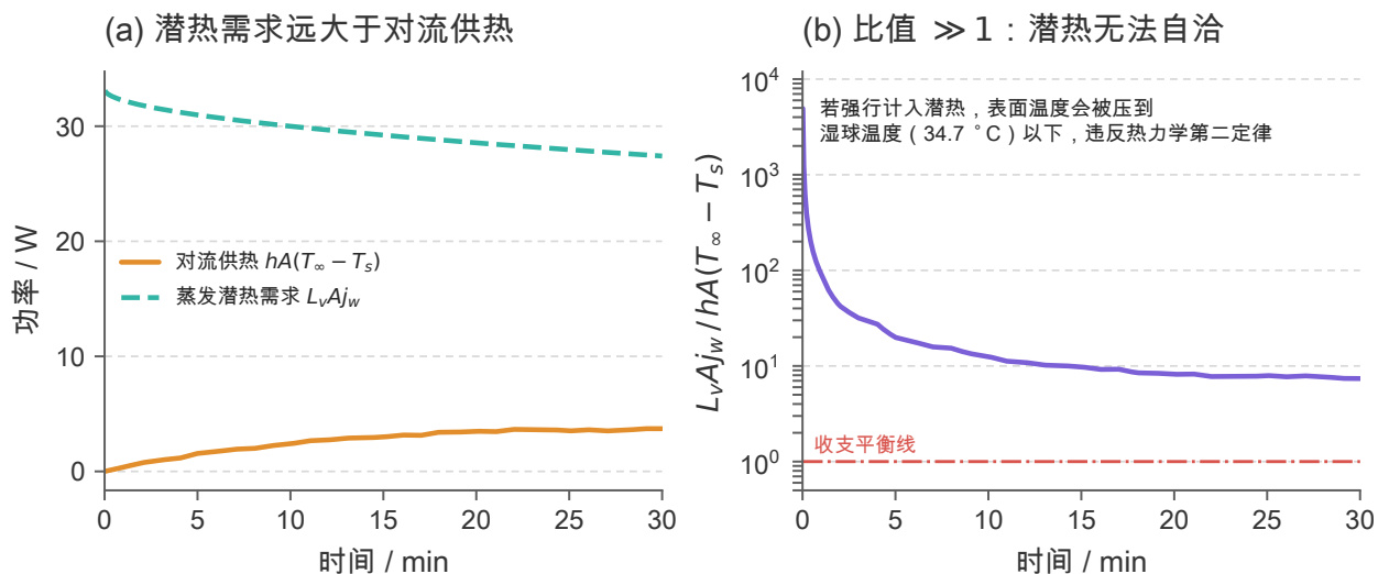
图1 蒸发潜热项的一致性检验：按题给 h_m 估算的潜热需求远大于对流供热能力，比值全程大于1，强行计入会把表面温度压到湿球温度以下，故题面参数体系对应忽略该项的简化（定量推导见附录B.1）。
