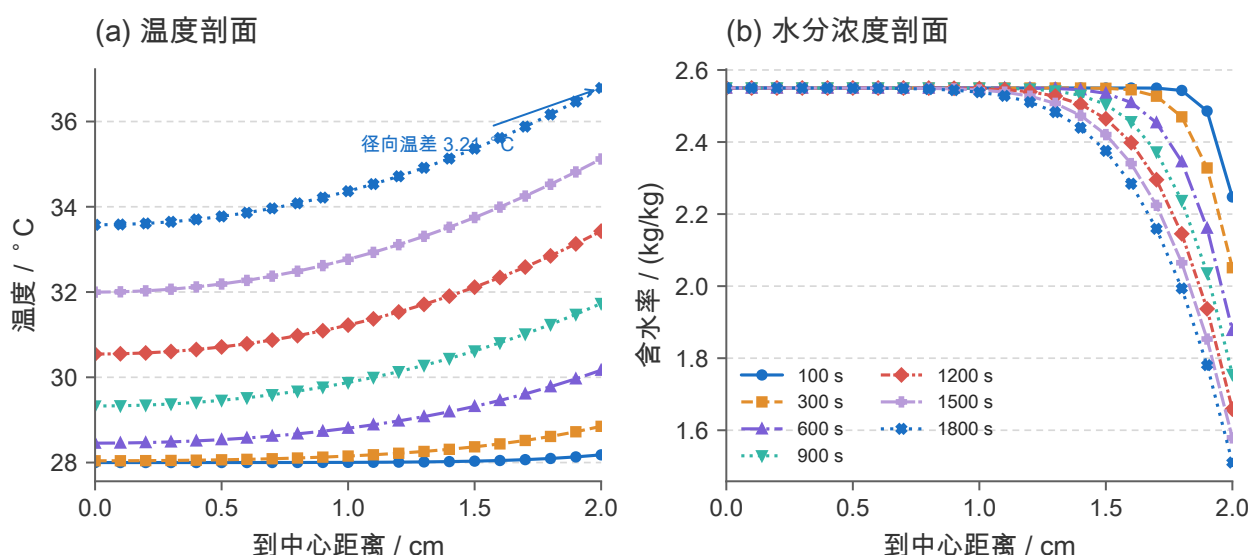
图 3 问题一若干时刻的径向剖面族：(a) 温度剖面，1800 s 时径向温差 3.21 ^{\circ}\text{C} ；(b) 水分浓度剖面，梯度集中在表面附近。
