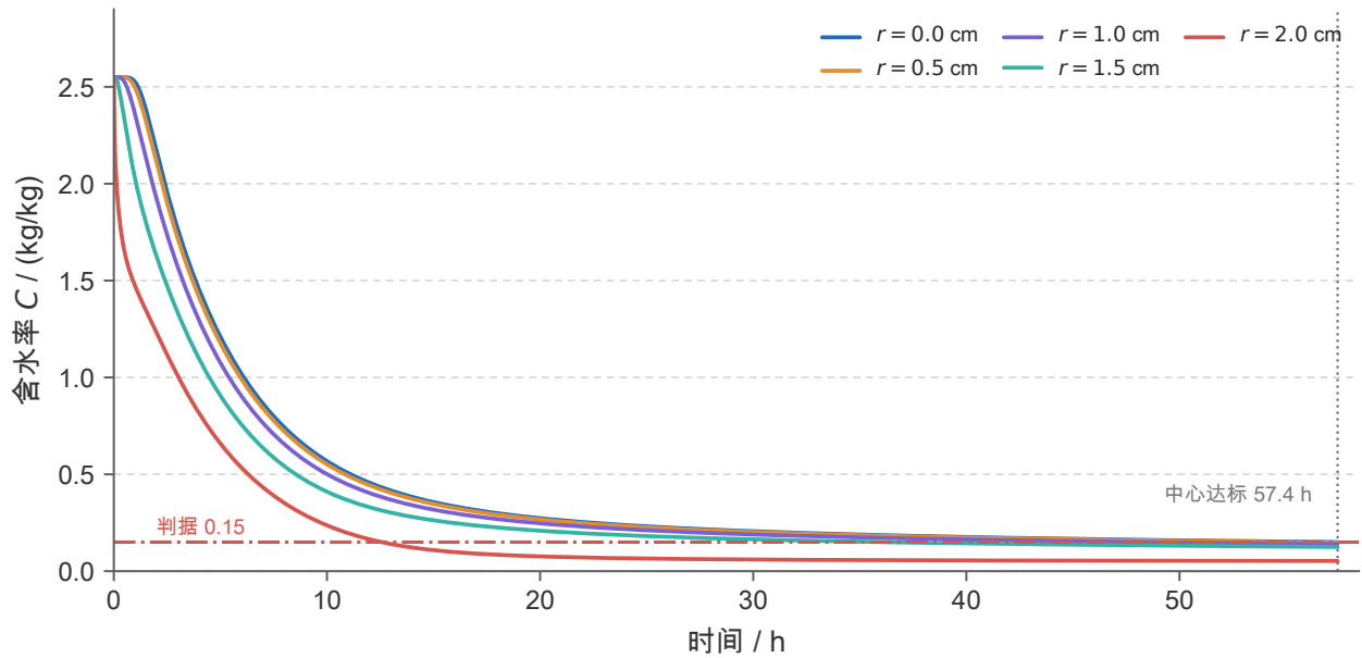
图 6 问题三 5 个径向位置的含水率历时曲线（ N = 200 、 \Delta t = 5 s）：中心最后达标（57.4 h），表面在 12.6 h 即低于判据，此后由于干壳控制。
