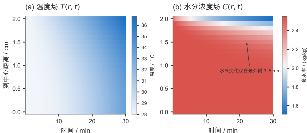
图 2 问题一的温度场 T(r, t) 与水分浓度场 C(r, t) ( N = 400 、 \Delta t = 1 \text{ s} )：30 min 内热量已接近穿透整个截面，而水分变化仅发生在最外侧 3 ~ 5 mm。
