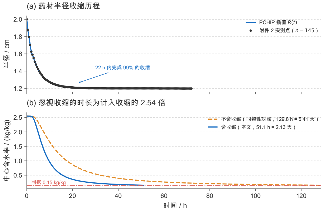
图 8 问题四：收缩历程与烘干时长的对照（附录 4 物性， N = 200 、 \Delta t = 5\text{ s} ）。(a) 附件 2 的实测半径（ n = 145 ，间隔 1800 s，实测点以散点示出）与保单调三次 Hermite 插值曲线；插值后 \dot{R} \leq 0 恒成立、无过冲。(b) 中心水分浓度随时间的变化：含收缩时 51.08 h 达标，固定半径的对照工况需 129.79 h，收缩使烘干时长缩短约 61%。两图均为确定性数值结果，不含统计误差。
