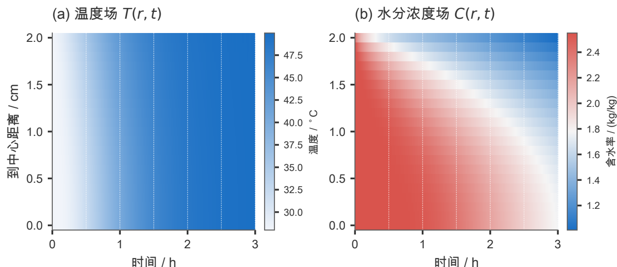
图4 问题二的温度场 T(r, t) 与水分浓度场 C(r, t) ( N = 200 、 \Delta t = 5 s)。温度在 1 h 内已接近均匀 (3 h 时径向温差仅 0.12^\circ\text{C} )，而水分浓度的高梯度区自表面向内推进：3 h 时表面已降到 1.0082\text{ kg/kg} ，中心仍有 1.7663\text{ kg/kg} ，变化尚未波及 r \lesssim 1.0\text{ cm} 以内的芯部。
