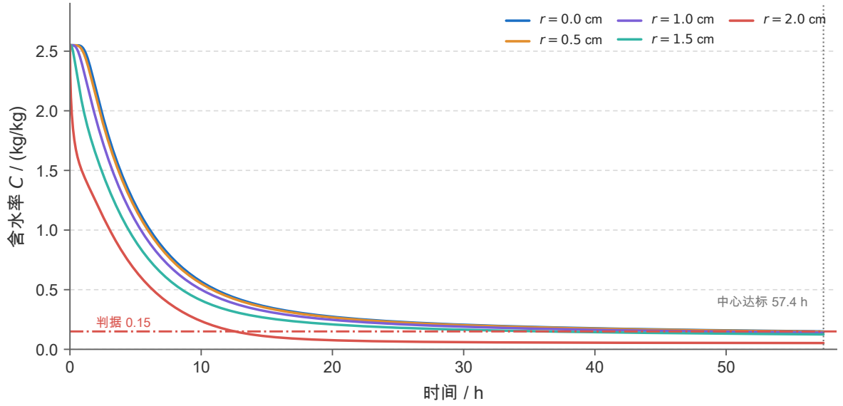
图6 问题三5个径向位置的含水率历时曲线 ( N = 200 、 \Delta t = 5 s)：中心最后达标 (57.4 h)，表面在12.6 h即低于判据，此后由于壳控制。
