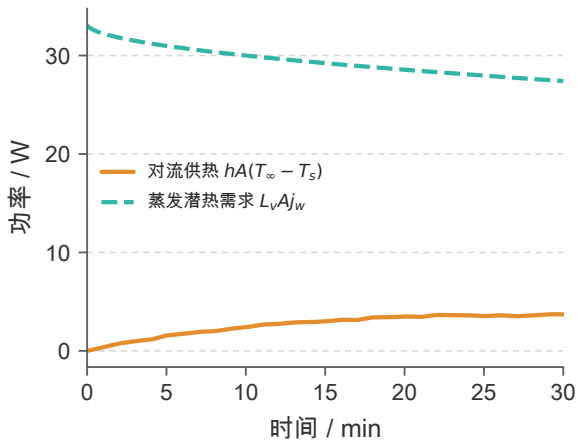
(a) 潜热需求远大于对流供热
