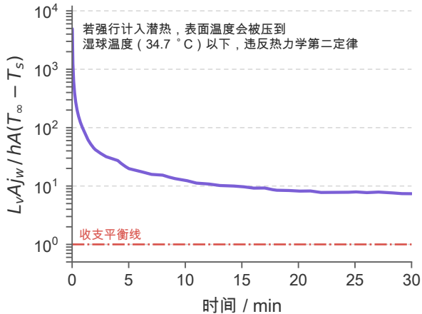
(b) 比值 \gg 1 : 潜热无法自洽
