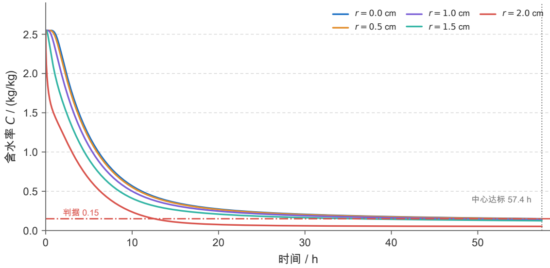
图6 问题三 5 个径向位置的含水率历时曲线 ( N = 200 、 \Delta t = 5 s)：中心最后达标 (57.4 h)，表面在 12.6 h 即低于判据，此后由于干壳控制。
