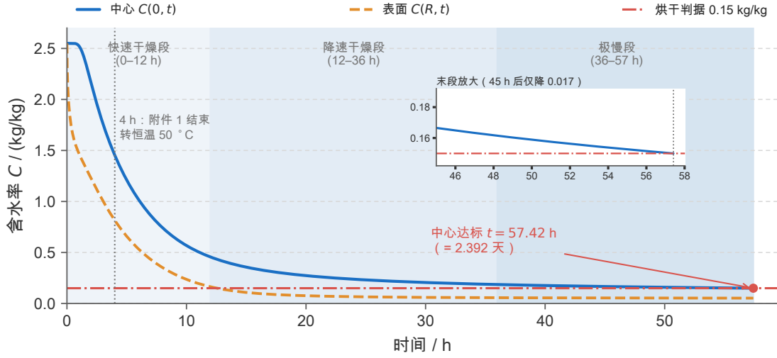
图 5 问题三干燥曲线：中心与表面水分浓度随时间的变化 ( N = 200 、 \Delta t = 5 s，判据为各点 C < 0.15 kg/kg)，右上角插图为 45 h 之后的放大。
