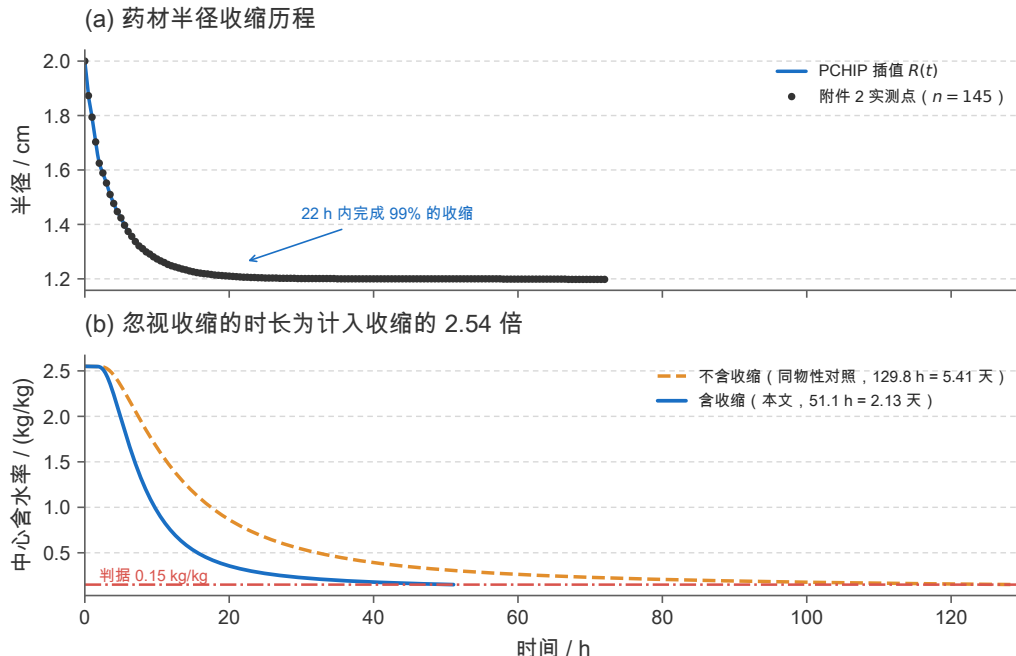
图 8 问题四: 收缩历程与烘干时长的对照 (附录 4 物性, N = 200 、 \Delta t = 5 s)。(a) 附件 2 的实测半径 ( n = 145 , 间隔 1800 s, 实测点以散点示出) 与保单调三次 Hermite 插值曲线; 插值后 \dot{R} \leq 0 恒成立、无过冲。(b) 中心水分浓度随时间的变化: 含收缩时 51.08 h 达标, 固定半径的对照工况需 129.79 h, 收缩使烘干时长缩短约 61%。两图均为确定性数值结果, 不含统计误差。
