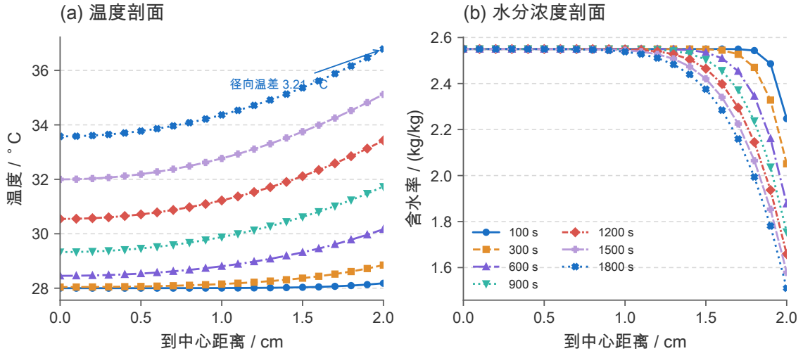
图 3 问题一若干时刻的径向剖面族：(a) 温度剖面，1800 s 时径向温差 3.21 ^{\circ}\text{C} ；(b) 水分浓度剖面，梯度集中在表面附近。
