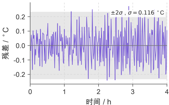
(c) 温度残差的时序
