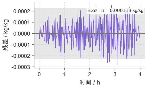
(d) 水分浓度残差的时序
