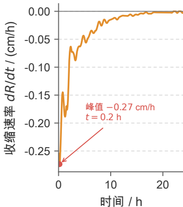
(b) 收缩速率 dR/dt
