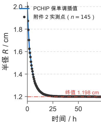
(a) 半径收缩历程
