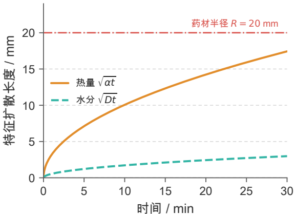
(a) 两个特征长度相差一个量级
