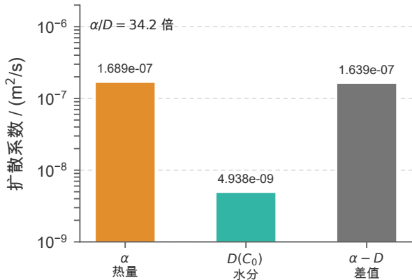
(b) 两个扩散系数相差 34 倍
